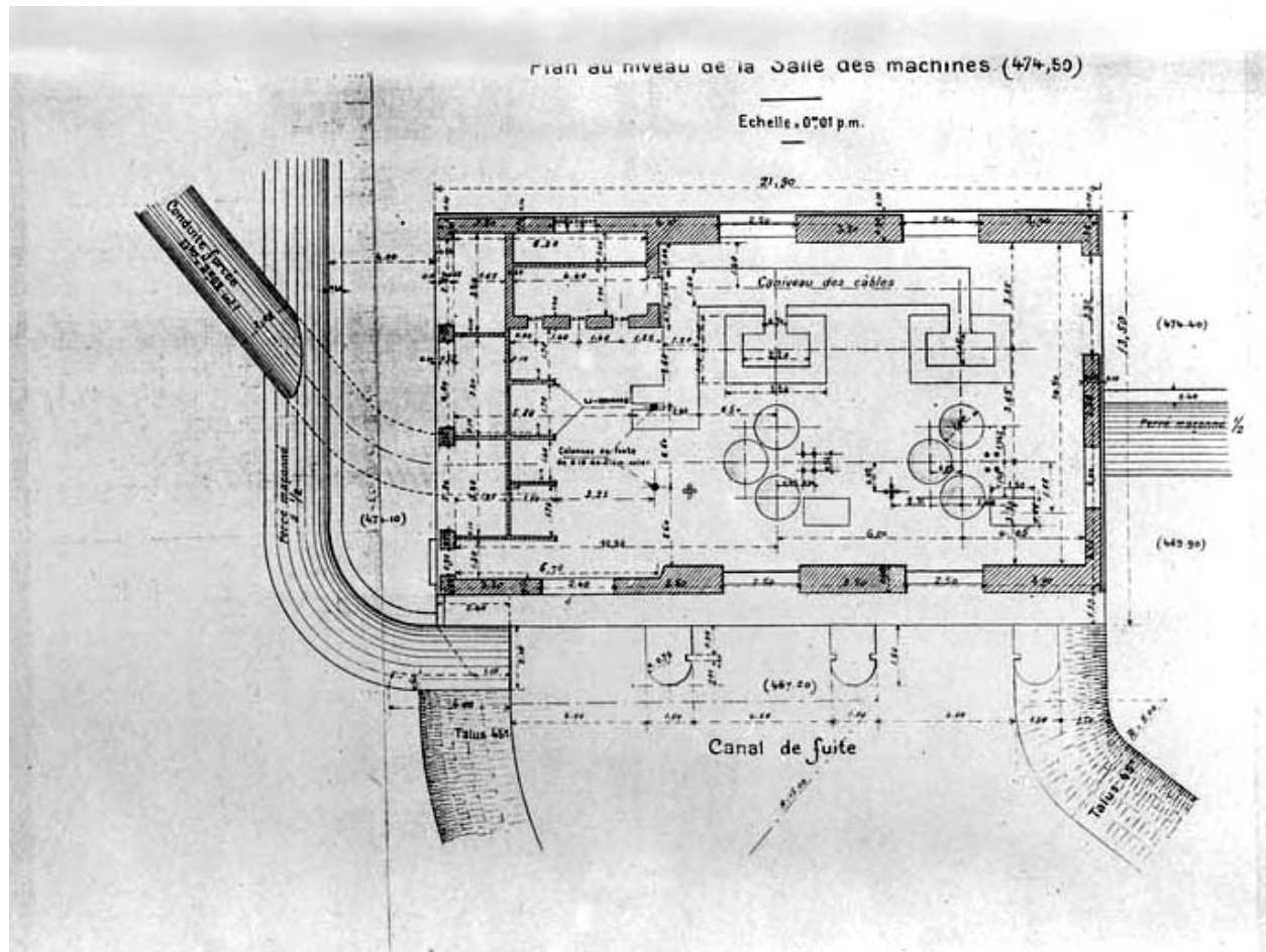
Usine du lac de Chalain. Bâtiment. Plan [détail] : Plan au niveau de la salle des machines.
