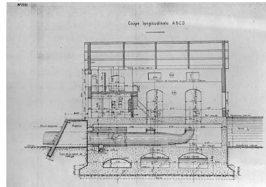
Usine du lac de Châlain. Bâtiment. Coupes [détail] : Coupe longitudinale ABCD. Phot. Jérôme Mongreville, Phot. Société générale d'Entreprises IVR43_19913900614V
