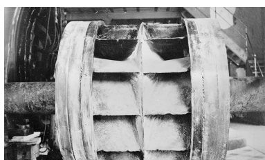
Turbine Francis double démontée : aubes de la roue. Phot. Jérôme Mongreville IVR43_19913900220X
