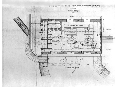
Usine du lac de Châlain. Bâtiment. Plan [détail] : Plan au niveau de la salle des machines. Phot. Jérôme Mongreville, Phot. Société générale d'Entreprises IVR43_19913900613V
