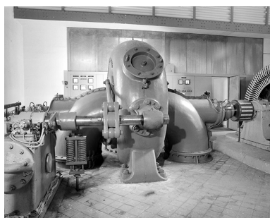
Intérieur de la centrale : turbine double Escher Wyss. Phot. Jérôme Mongreville IVR43_19913900622X
