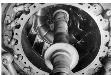
Turbine Francis double : cercle de vannage et directrices. Phot. Jérôme Mongreville IVR43_19913900221X
