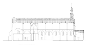
coupe longitudinale sur l'église IVR26_20122100226A1YY
