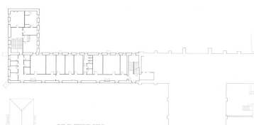
plan du troisième niveau IVR26_20122100225A0YY
