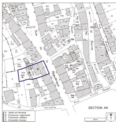
Plan-masse et de situation. Extrait du plan cadastral, 1980, section AI, échelle 1:1000. Dess. André Céréza IVR43_20093900299NUDA
