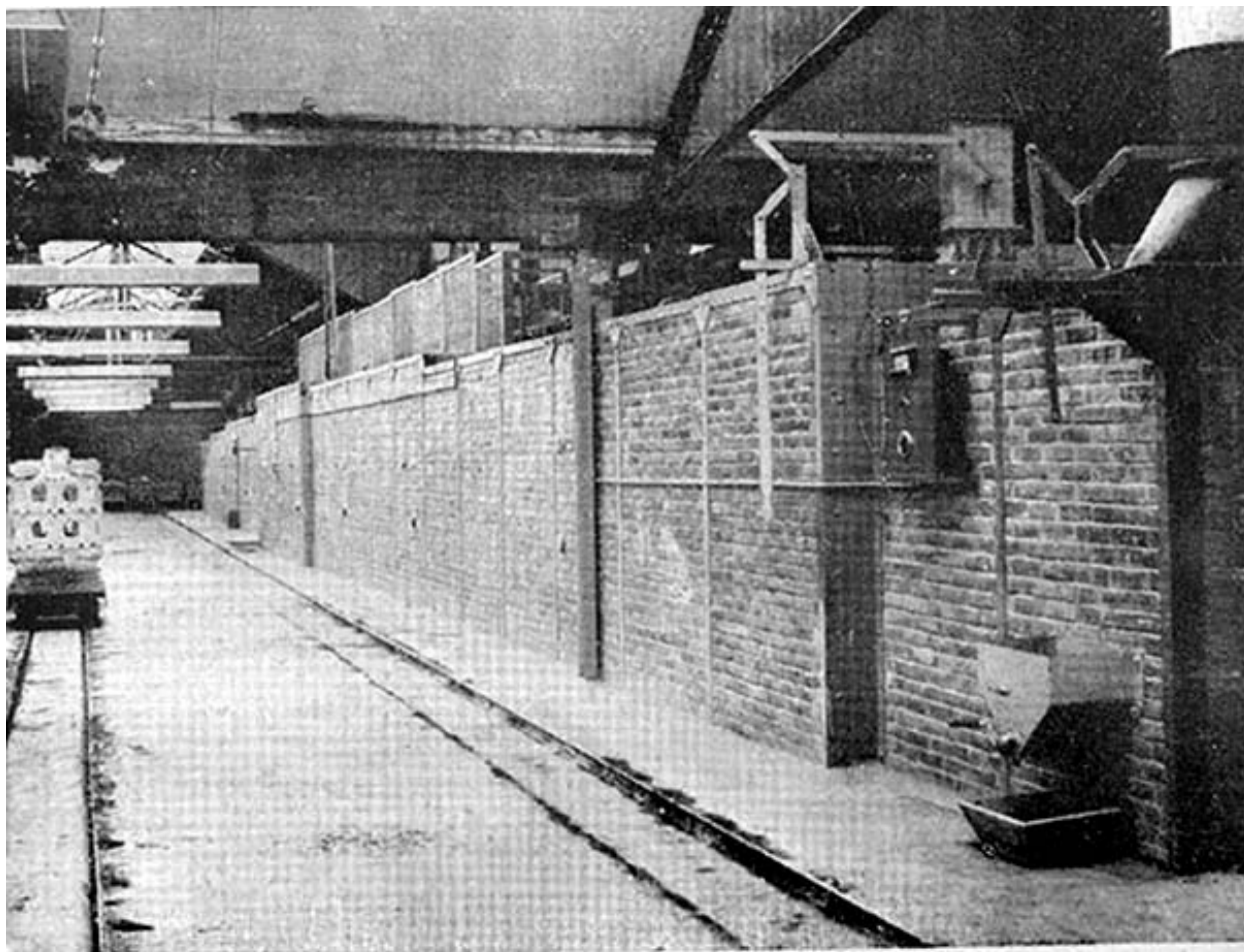
Four électrique tunnel pour la cuisson de l'émail à 1.400°
