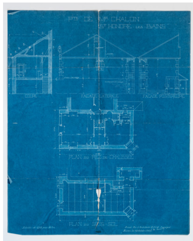
Plans, coupe et élévations de la pharmacie.
