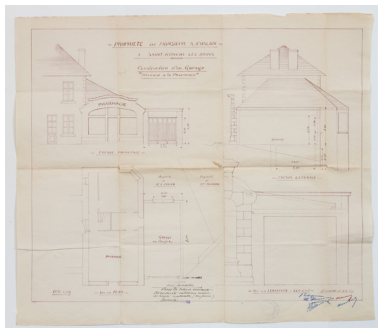
Plan et élévations du garage attenant à la pharmacie. Phot. Pierre-Marie Barbe- Richaud, Autr. auteur inconnu IVR26_20195800339NUC2A
