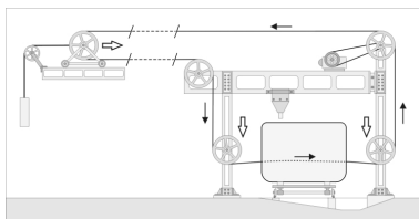
Schéma de fonctionnement. Dess. André Céréza IVR43_20013900835NUDY
