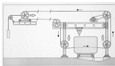
Schéma de fonctionnement. Phot. Yves Sancey, Autr. André (dessinateur) NEPASUTILISERCéréza IVR43_19993900021ZA
