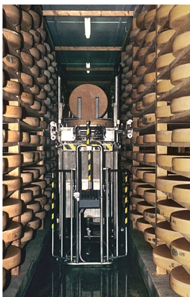
Robot de retournement et de salage des meules de comté. Phot. Jérôme Mongreville IVR43_19953900290ZA
