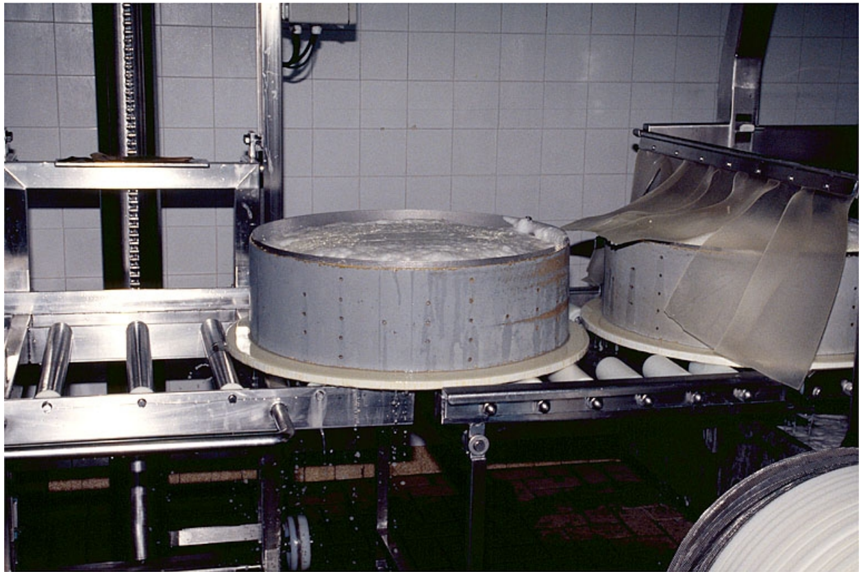
Moules remplis de caillé sortant du soutirage sous vide.
