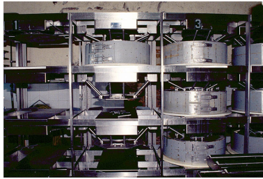
Moules dans la presse hydraulique. Phot. Jérôme Mongreville IVR43_19953900249ZA
