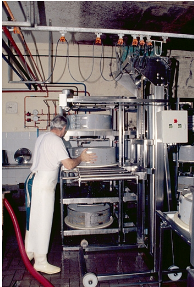
Mise en place d'un moule dans la presse hydraulique. Phot. Jérôme Mongreville IVR43_19953900246ZA
