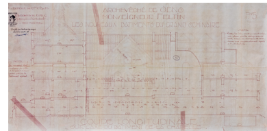
Coupe des nouveaux bâtiments du grand séminaire, 1934. Phot. Pierre-Marie Barbe-Richaud, Autr. Lazare Bertrand IVR26_20238901048NUC2A
