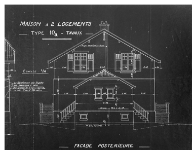
Elévation de la façade postérieure. Phot. Jérôme Mongreville IVR43_19893900433X
