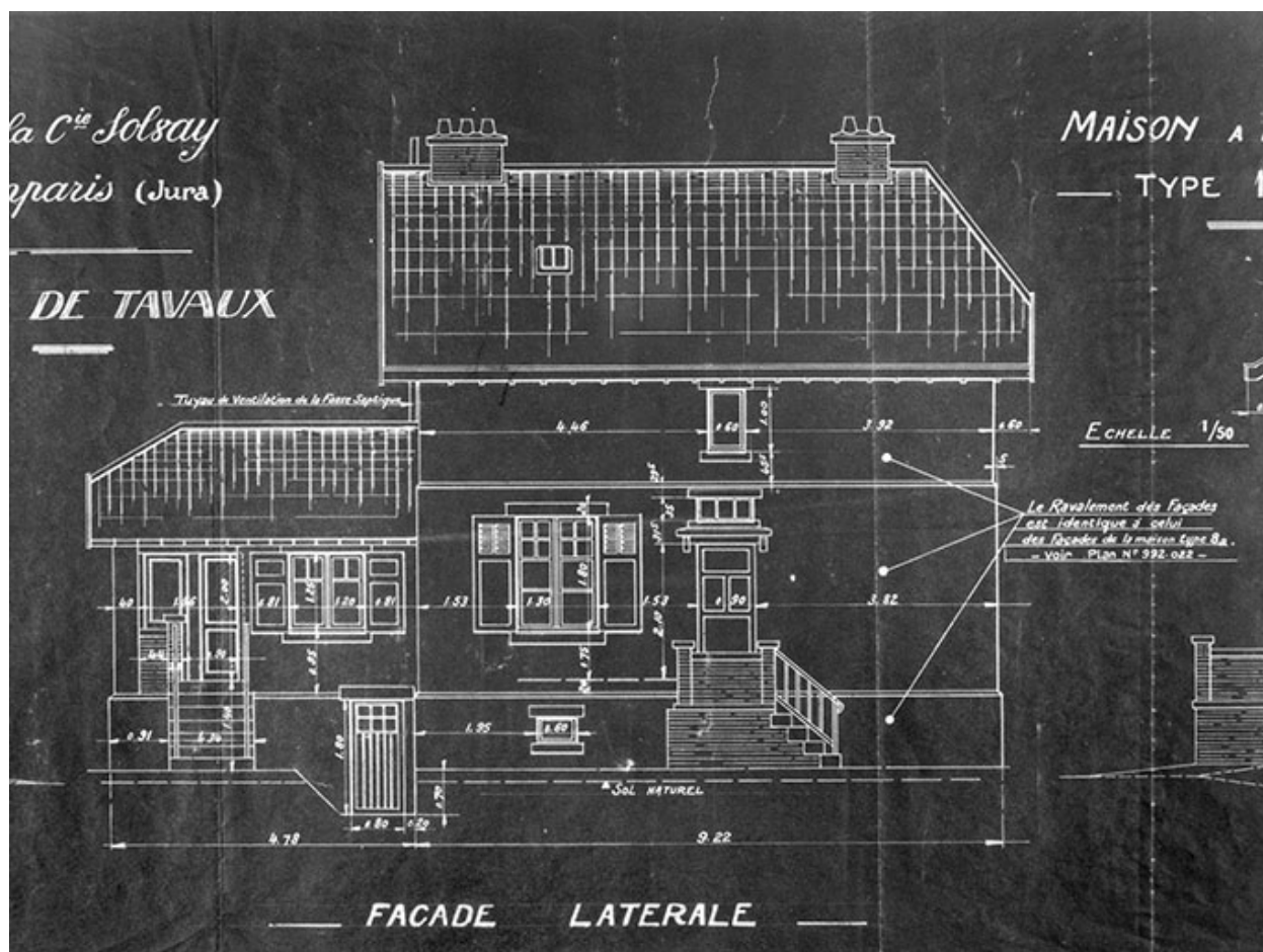
Elévation de la façade latérale.
