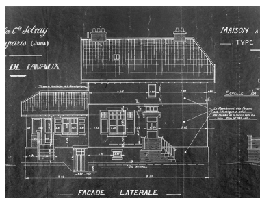
Elévation de la façade latérale. Phot. Jérôme Mongreville IVR43_19893900432X
