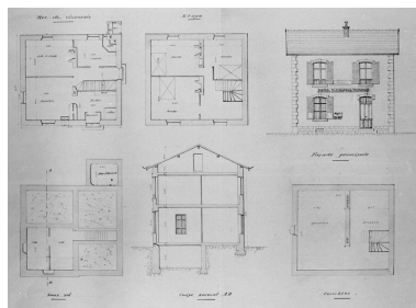
[Projet type de bureau de poste : plans, coupe et élévation]. Phot. Jérôme Mongreville IVR43_19973900283X
