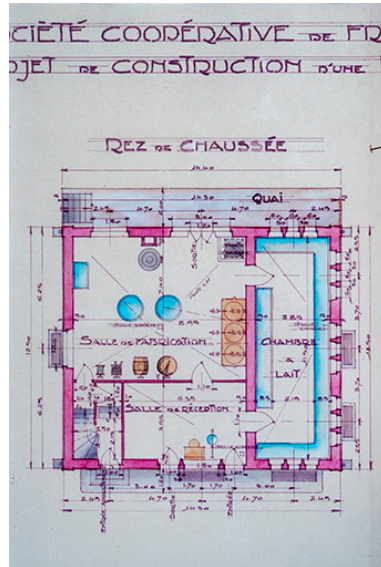
Société coopérative de fromagerie. Avant-projet de construction d'une fruitière - Plan du rez-de-chaussée, 1929. Phot. Jérôme Mongreville IVR43_20182500123NUC4A
