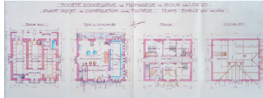
Société coopérative de fromagerie. Avant-projet de construction d'une fruitière - Plans, 1929. Phot. Jérôme Mongreville IVR43_20182500122NUC4A
