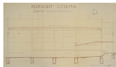
Modern-Cinéma. Coupe longitudinale. S.d. [1936]. Phot. Jérôme Mongreville IVR43_20223900362NUC4A
