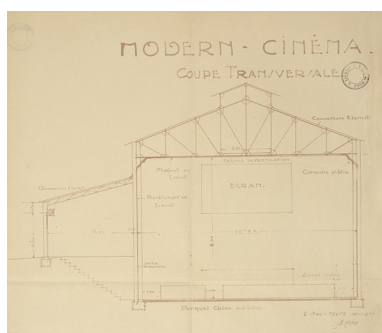
Modern-Cinéma. Coupe transversale. S.d. [1936]. Phot. Jérôme Mongreville IVR43_20223900360NUC4A
