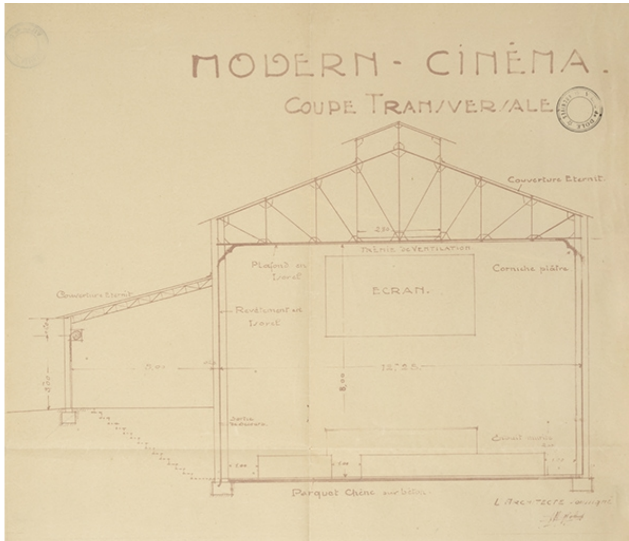
Modern-Cinéma. Coupe transversale. S.d. [1936].
