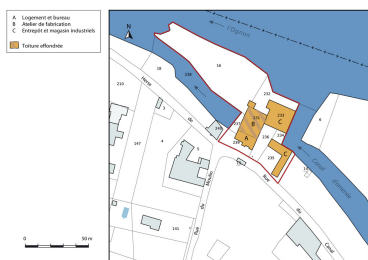
Plan-masse et de situation. Extrait du plan cadastral, 2015, section AB. Dess. Mathias Papigny IVR43_20152502659NUDA
