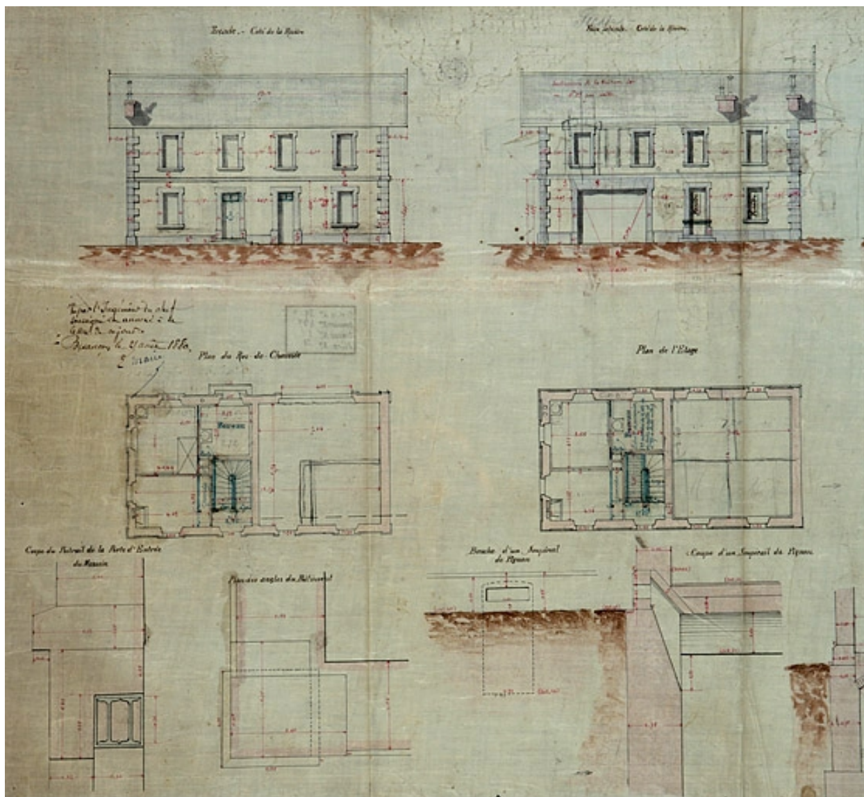
[Projet de maison d'éclusier sur l'île de Tarragnoz : plans et élévations], 1880.
