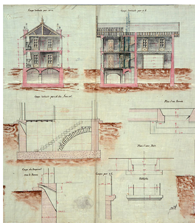
[Projet de maison d'éclusier sur l'île de Tarragnoz : coupes], 1880. Phot. Yves Sancey, Autr. Rascol IVR43_20062500050NUCA
