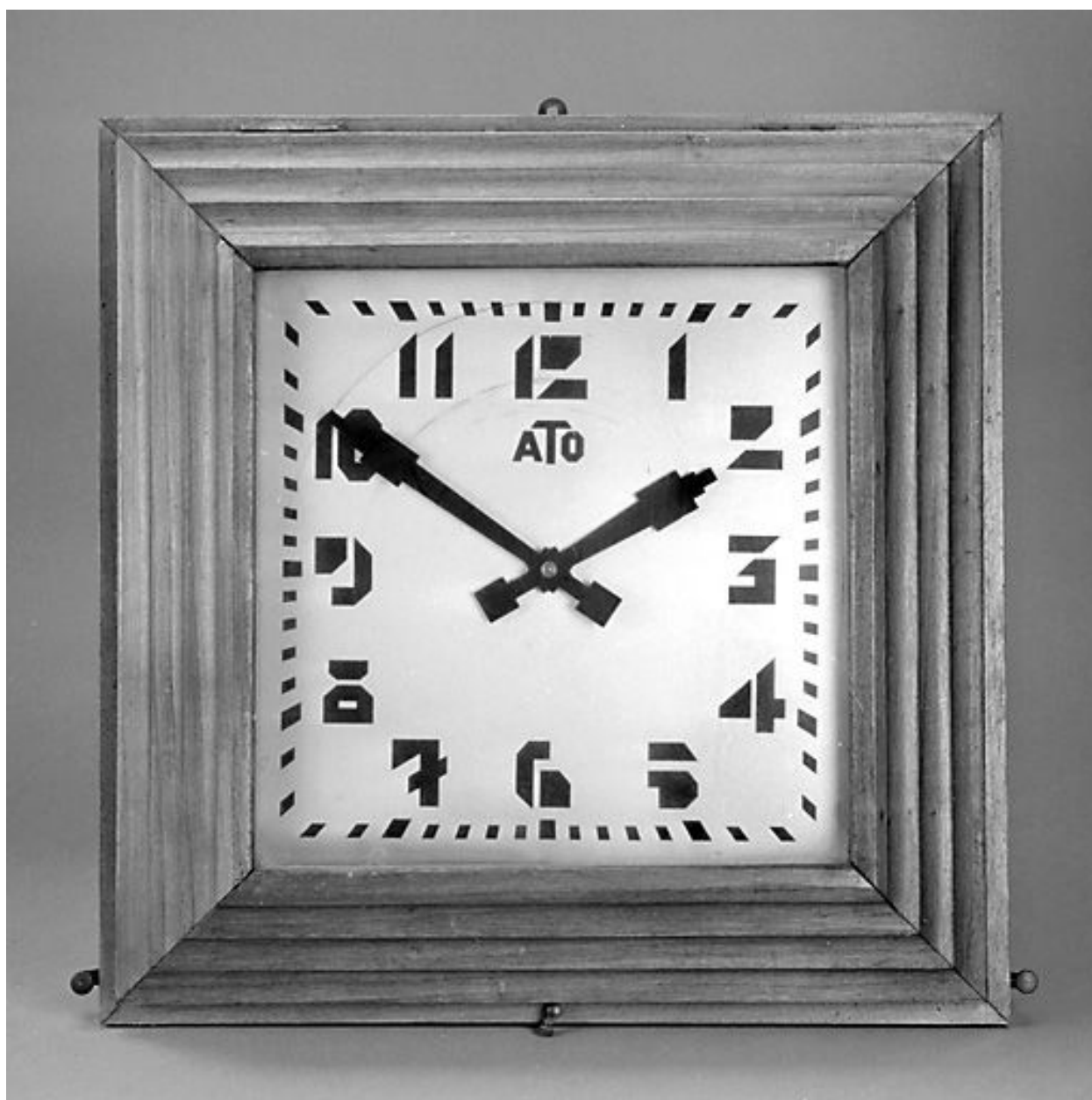
Horloge électrique Ato. Horloge secondaire (école professionnelle dite Ecole nationale d'Optique puis lycée polyvalent Victor Bérard, Morez).
