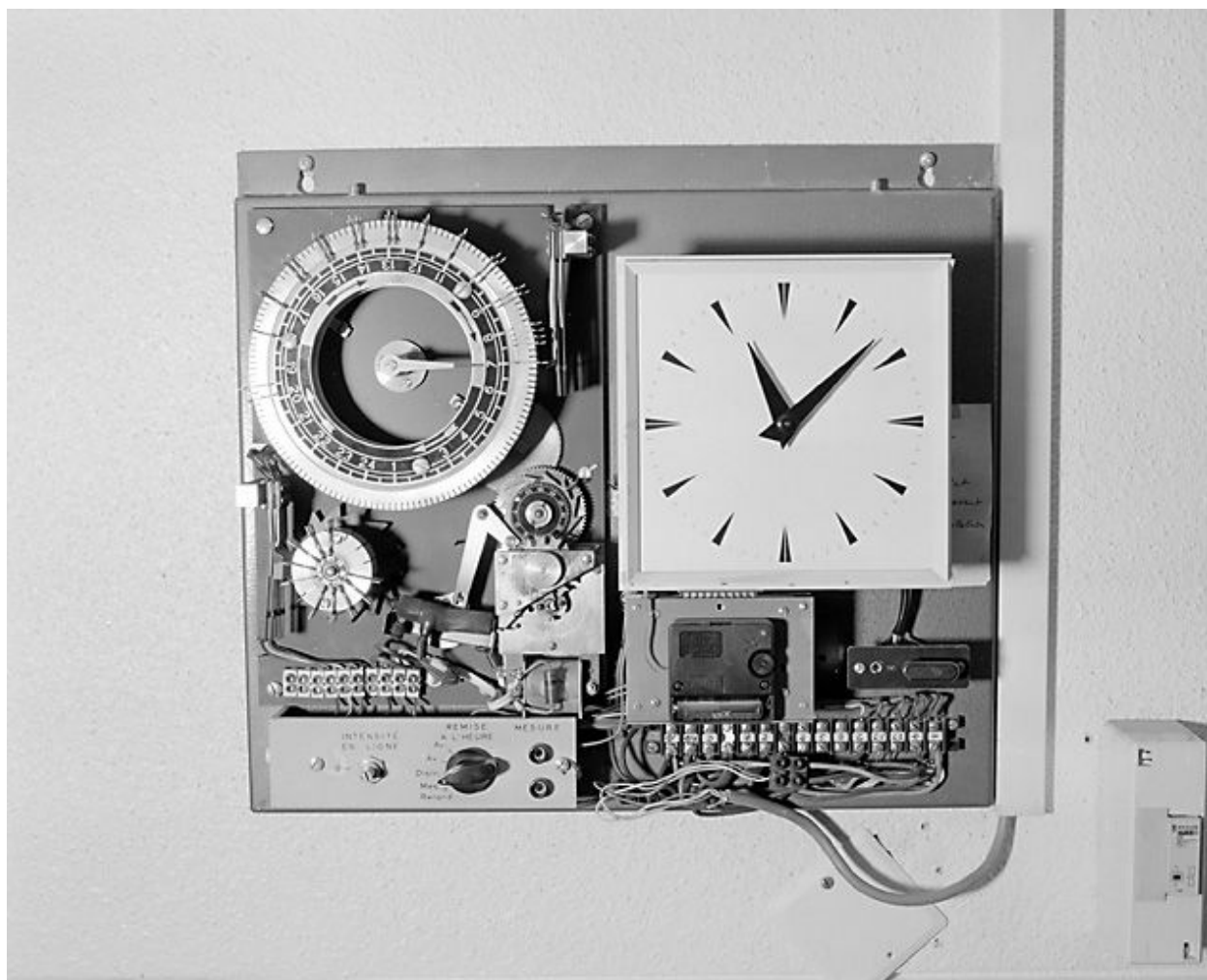
Horloge électrique Ato. Horloge mère : modules sonnerie et garde-temps (école professionnelle dite Ecole nationale d'Optique puis lycée polyvalent Victor Bérard, Morez).
