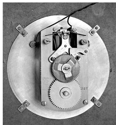
Horloge électrique Ato. Horloge secondaire : système moteur (école professionnelle dite Ecole nationale d'Optique puis lycée polyvalent Victor Bérard, Morez). Phot. Jérôme Mongreville IVR43_20023900148X
