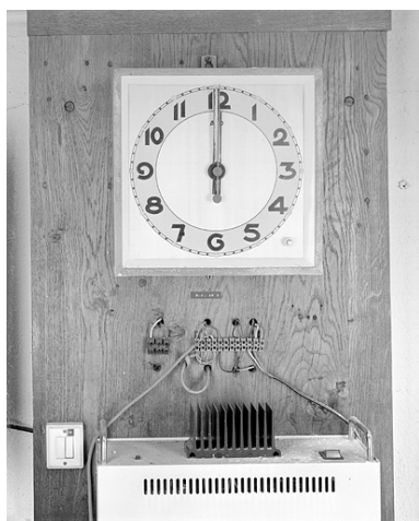
Horloge électrique Ato (Observatoire de Besançon, la Bouloie). Phot. Jérôme Mongreville IVR43_20032500686V
