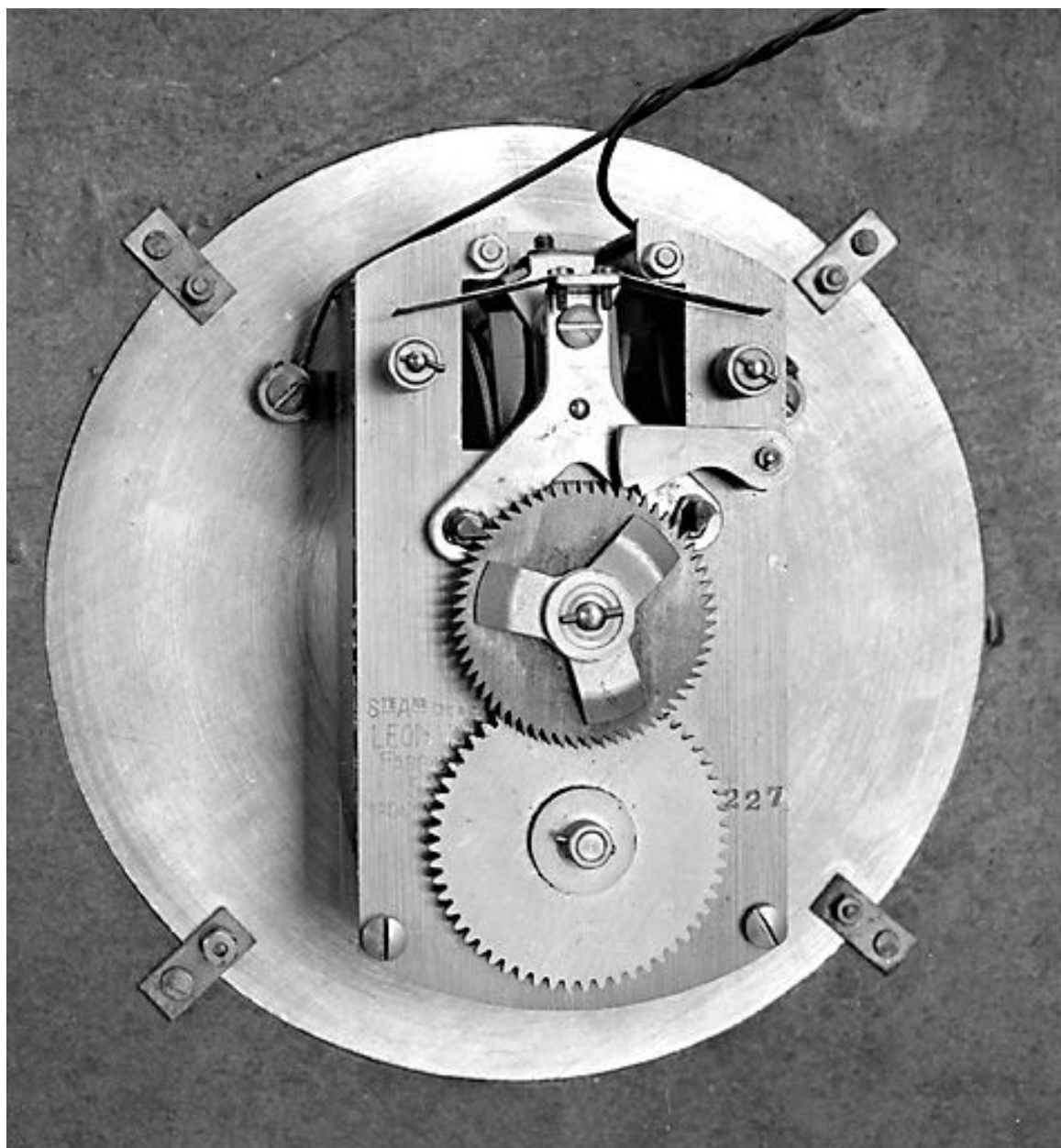
Horloge électrique Ato. Horloge secondaire : système moteur (école professionnelle dite Ecole nationale d'Optique puis lycée polyvalent Victor Bérard, Morez).
