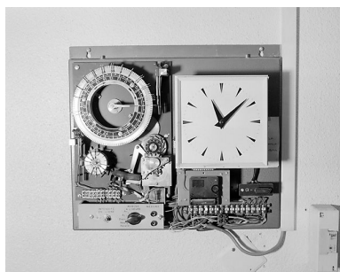
Horloge électrique Ato. Horloge mère : modules sonnerie et garde-temps (école professionnelle dite Ecole nationale d'Optique puis lycée polyvalent Victor Bérard, Morez). Phot. Jérôme Mongreville IVR43_20023900149X
