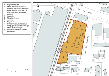
Plan-masse et de situation. Extrait du plan cadastral, 2019. Dess. Bertrand Turina IVR43_20192501141NUDA
