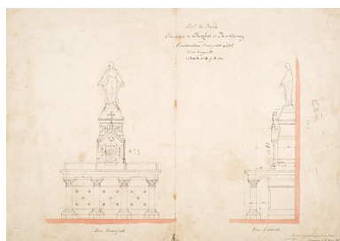
Communes de Chazelot et Montferney. Construction d'un petit autel. Dessin d'ensemble. 23 mars 1872. Phot. Jérôme Mongreville, Autr. Ferréol François Just Alfred Ducat IVR43_20112500237NUC4A
