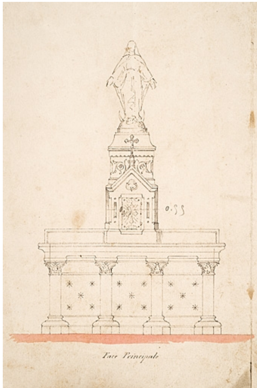
Communes de Chazelot et Montferney. Construction d'un petit autel. Dessin d'ensemble. [Détail :] Face principale. 23 mars 1872.
