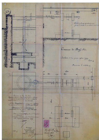
Installation de deux pompes système Japy. 1907.
