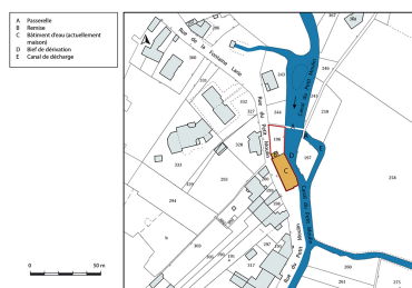
Plan-masse et de situation. Extrait du plan cadastral, 2019. Dess. Bertrand Turina IVR43_20197000215NUDA
