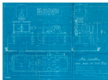
Plan d'installation d'une pompe. [début du 20e siècle]. Repro. Jérôme Mongreville, Autr. auteur inconnu IVR43_20197000009NUC4A
