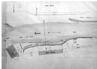
Construction d'un mur [...] Plan et coupe transversale. Phot. Jérôme Mongreville, Autr. Bonnefoy IVR43_19943900432X
