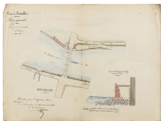
Pont de Pontailler. Plan général. Projet d'une banquette de halage. 1872. Phot. Thierry Kuntz IVR26_20172100158NUC4A
