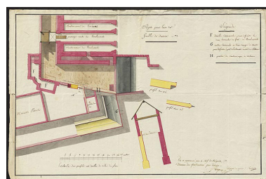
Projet pour l'an 10 [-casemate pour défendre]. An 10 [1801-1802]. Autr. auteur inconnu IVR43_20252500011NUC4A
