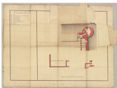
Fol. 18 Château de Blamont : plans (magasin pour 10,000 milliers de poudre) [vue 4]. Autr. auteur inconnu IVR43_20242500027NUC4A
