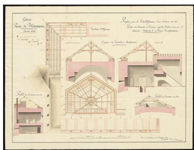
Projet pour le rétablissement d'une toiture sur les parties des casernes à l'épreuve dont les voûtes n'ont pas été détruites. 1819.
