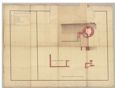
Fol. 18 Château de Blamont : plans (magasin pour 10,000 milliers de poudre) [vue 3]. Autr. auteur inconnu IVR43_20242500026NUC4A
