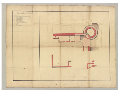
Fol. 18 Château de Blamont : plans (magasin pour 10,000 milliers de poudre) [vue 1]. Autr. auteur inconnu IVR43_20242500024NUC4A
