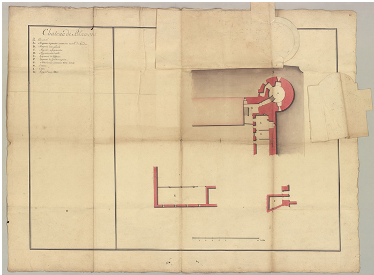
Fol. 18 Château de Blamont : plans (magasin pour 10,000 milliers de poudre) [vue 4].
