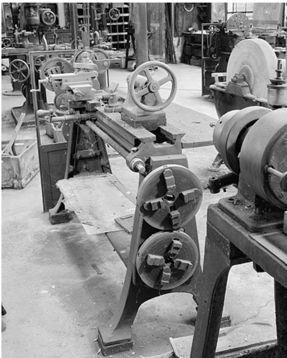
Vue de la vis-mère et du traînard.
