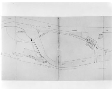
Suppression de l'usine Thévenin Zéphirin de Morez [...] Plan des lieux [détail]. Dessin, 1920. Echelle 1:500. Phot. Jérôme Mongreville IVR43_19993900511V
