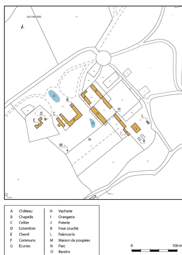
Plan-masse et de situation, extrait du plan cadastral (2020). Dess. Pierre-Marie Barbe-Richaud IVR26_20205800633NUDA
