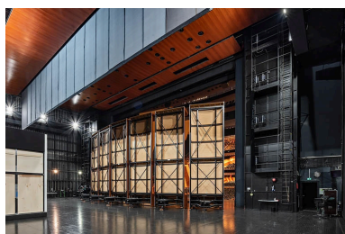
Maîtrise de l'acoustique : réflecteurs acoustiques vus de dos, depuis la scène. Phot. Pierre-Marie Barbe-Richaud IVR26_20212100128NUC4A
