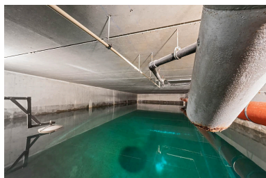
Bassin en sous-sol (500 m3). Phot. Pierre-Marie Barbe-Richaud IVR26_20212100166NUC4A
