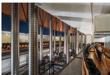
Avant-scène : colonnes Spiralift soutenant le plancher de la fosse d'orchestre. A droite et à gauche, rangées de sièges supplémentaires. Phot. Pierre-Marie Barbe-Richaud IVR26_20212100149NUC4A
