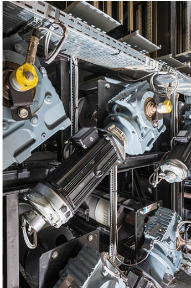
Equipes contrebalancées : moteurs électriques. Phot. Pierre-Marie Barbe-Richaud IVR26_20212100145NUC4A
