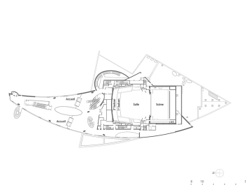
Plan au 3e étage (niveau 12,60 m). D'après un plan non daté fourni par l'Opéra de Dijon. Dess. Aline Thomas IVR26_20232100057NUDA
