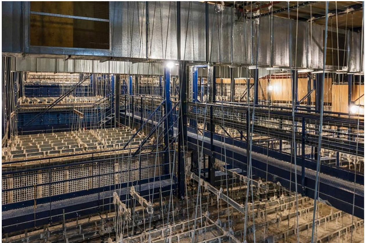
Maîtrise de l'acoustique : fixation du plafond de la salle.
