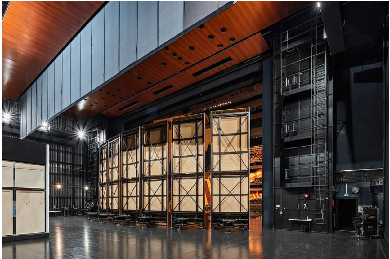
Maîtrise de l'acoustique : réflecteurs acoustiques vus de dos, depuis la scène.
