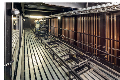
Cage de scène : gril avec poules de renvoi et fils. Phot. Pierre-Marie Barbe-Richaud IVR26_20212100141NUC4A
