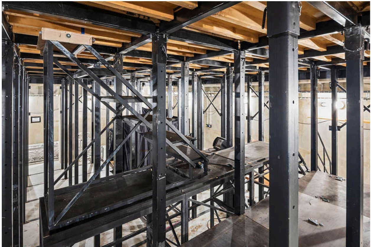
Cage de scène : dessous avec escalier mobile permettant aux acteurs d'apparaître sur scène via une trappe.
