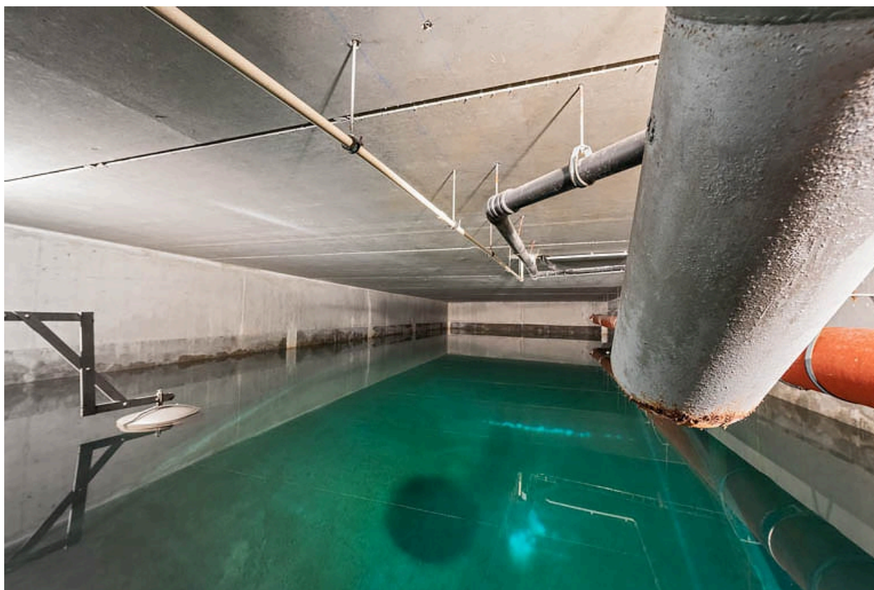
Bassin en sous-sol (500 m3).
