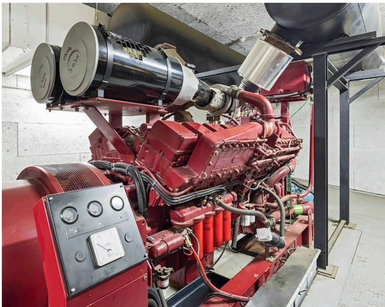
Groupe électrogène de secours (détail).
