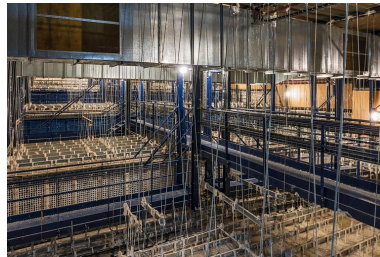
Maîtrise de l'acoustique : fixation du plafond de la salle. Phot. Pierre-Marie Barbe-Richaud IVR26_20212100176NUC4A
