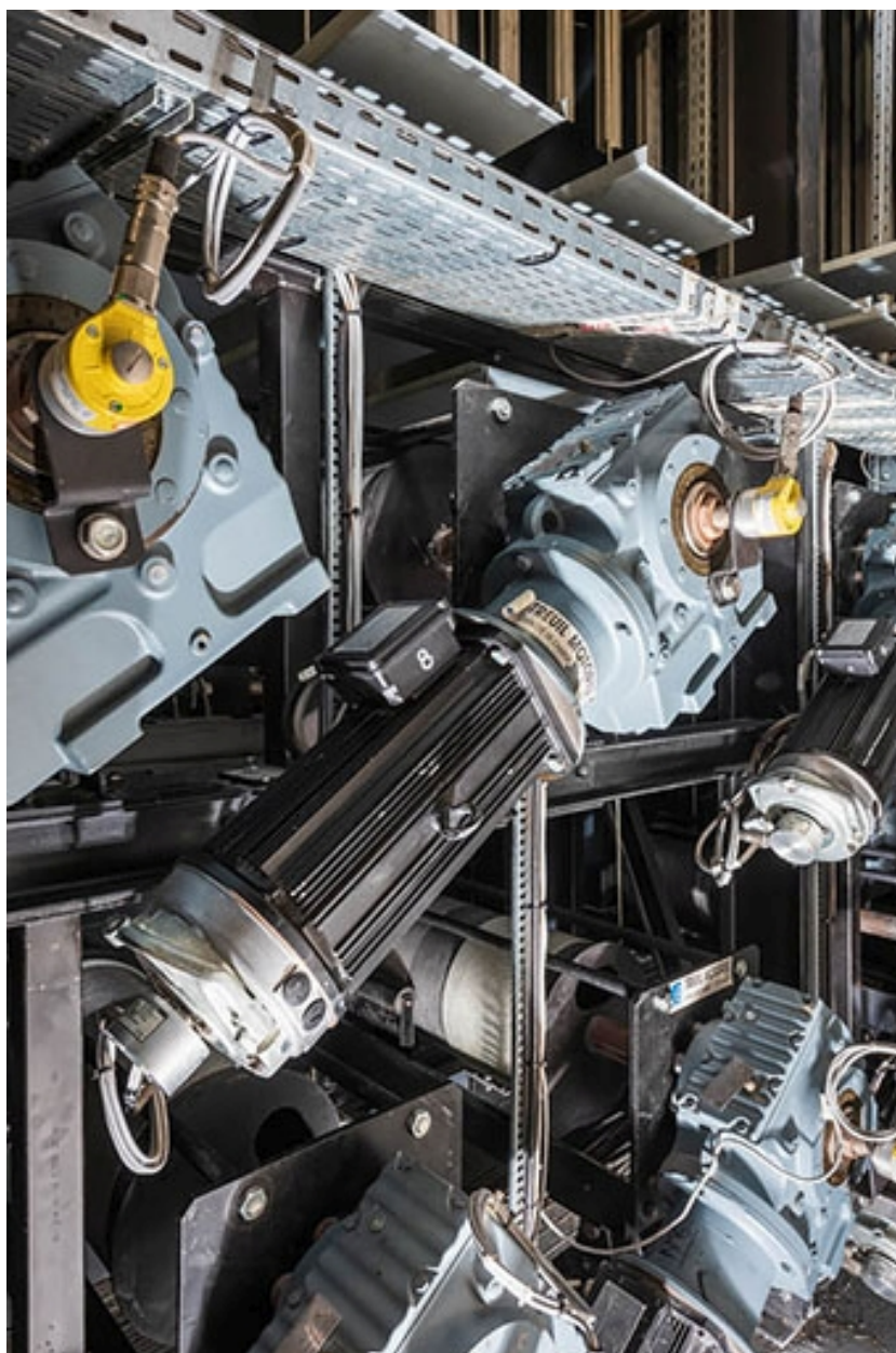
Equipes contrebalancées : moteurs électriques.
