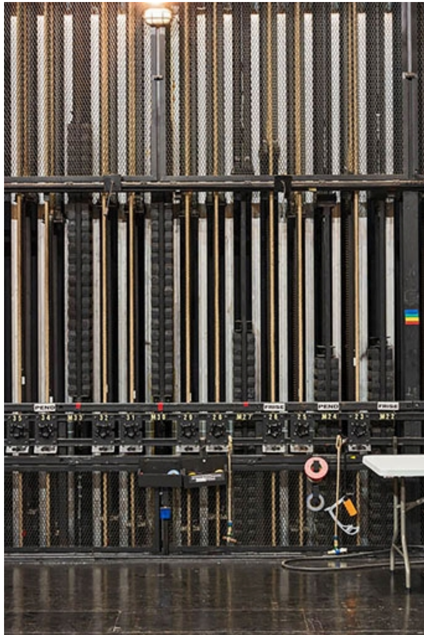
Cage de scène : fils de commande des perches et contrepoids ("équipe contrebalancée").
