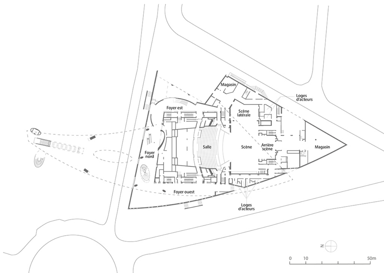
Plan au rez-de-chaussée (niveau 1,20 m). D'après un plan non daté fourni par l'Opéra de Dijon.
