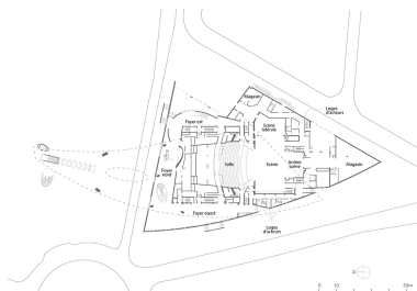
Plan au rez-de-chaussée (niveau 1,20 m). D'après un plan non daté fourni par l'Opéra de Dijon. Dess. Aline Thomas IVR26_20232100056NUDA
