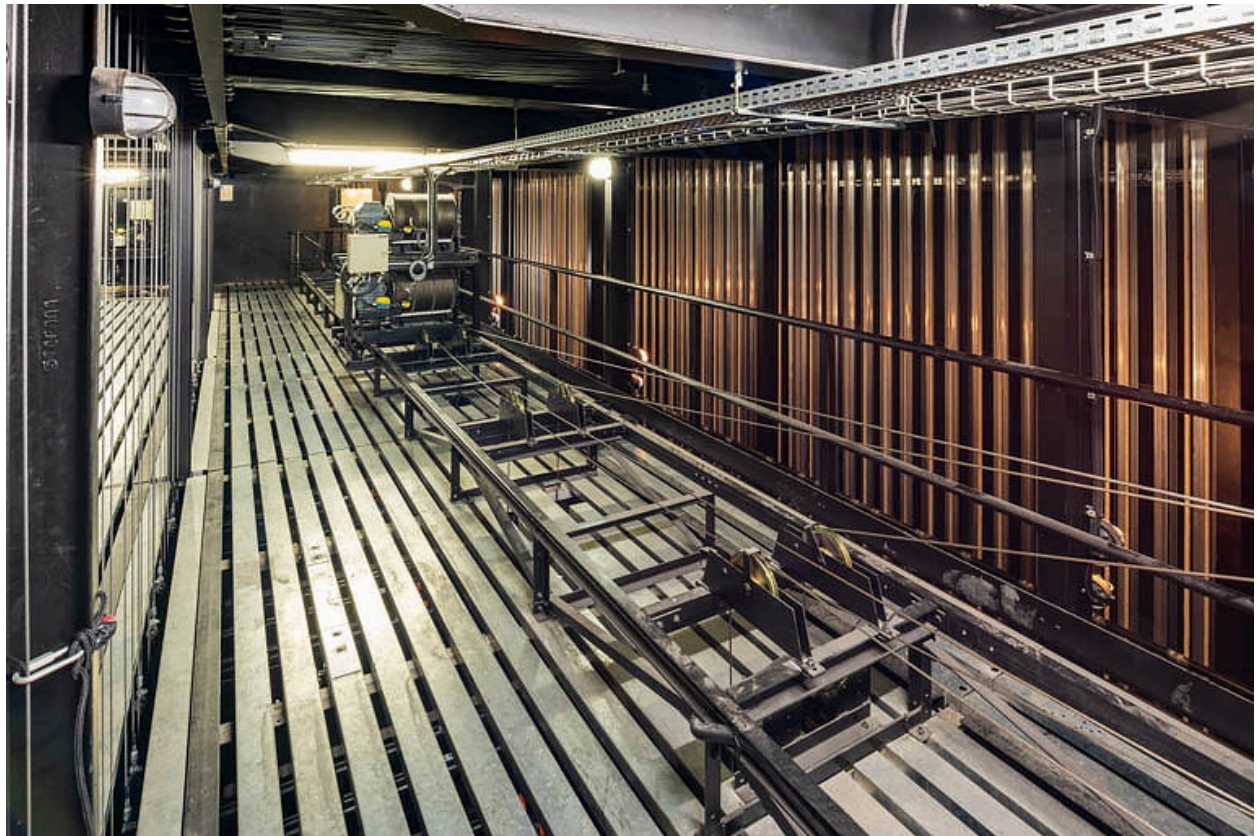
Cage de scène : gril avec poulies de renvoi et fils.
