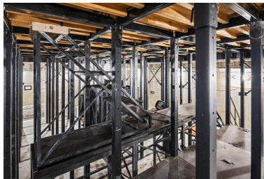
Cage de scène : dessous avec escalier mobile permettant aux acteurs d'apparaître sur scène via une trappe. Phot. Pierre-Marie Barbe-Richaud IVR26_20212100168NUC4A
