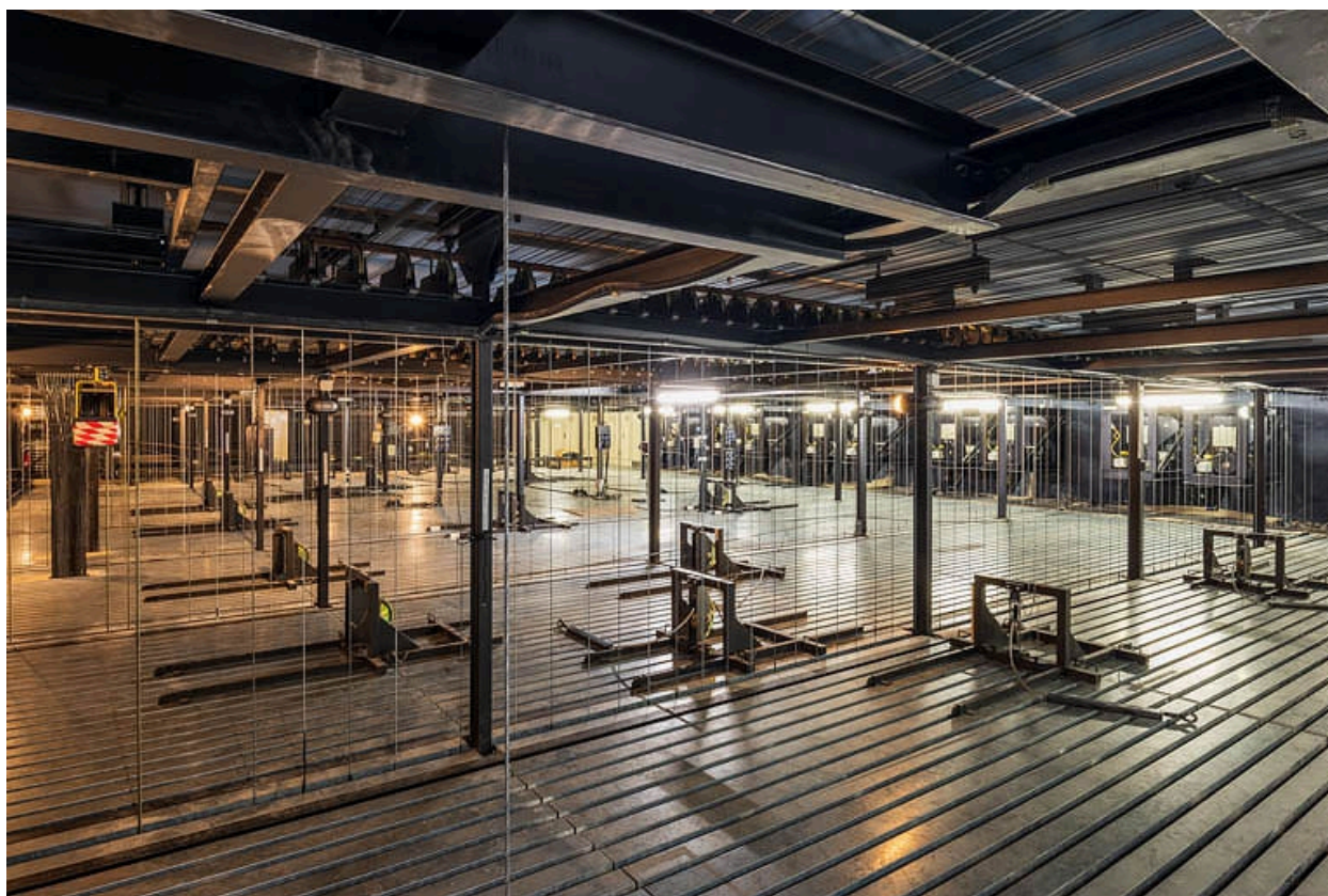
Cage de scène : gril.
