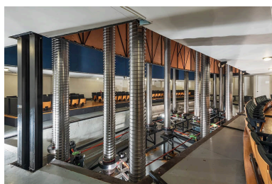
Avant-scène : colonnes Spiralift soutenant le plancher de la fosse d'orchestre. Phot. Pierre-Marie Barbe-Richaud IVR26_20212100148NUC4A
