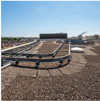
Toit terrasse au-dessus de la salle : rail du chariot permettant le déplacement de la nacelle utilisée pour le nettoyage des façades. Phot. Pierre-Marie Barbe-Richaud IVR26_20212100161NUC2A
