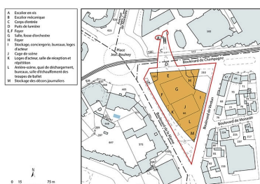
Plan-masse et de situation. Source : Direction générale des Finances Publiques - Cadastre ; mise à jour 2021, section BL, 1/1 000 réduit à 1/1 500. Dess. Aline Thomas IVR26_20222100079NUDA
