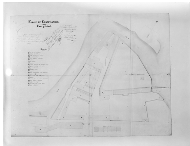
Forge de Champagnole - Plan général. Phot. Yves Sancey, Autr. J.-F. Borne IVR43_19973901995V
