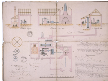
Plan, élévations et coupe du haut fourneau d'Autrey, ainsi que de la machine soufflante [...]. Phot. Yves Sancey, Phot. B. Besancenot IVR43_19877000017XA
