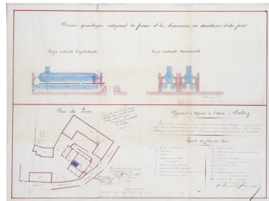
Plan et dessins géométriques annexés à la demande de M.M. Huot frères du 15 juin 1855 à l'effet d'obtenir l'autorisation de poser 2 chaudières et 2 machines à vapeur [...]. Phot. Yves Sancey IVR43_19907000140VA
