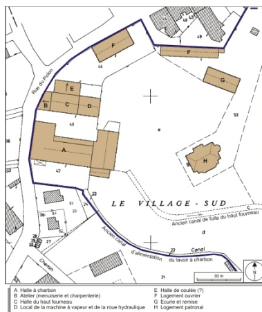
Plan-masse et de situation. Extrait du plan cadastral numérisé, 2008, section AD, 1:1000. Source : Direction générale des Finances Publiques - Cadastre ; mise à jour : 2008. Dess. André Céréza IVR43_20087000988NUDA
