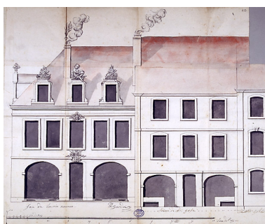
Elévation de la façade principale sur rue.
