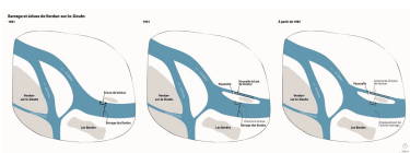
Plans schématiques (en 1841, 1931 et dès 1987) du barrage et de l'écluse de Verdun-sur-le-Doubs, échelle 1 / 5 000e. Dess. Aline Thomas IVR26_20227100071NUDA
