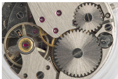
Détail : de gauche à droite, balancier-spiral, rochet et roue de couronne (côté ponts). Phot. Sonia Dourlot IVR43_20152500010NUC4A
