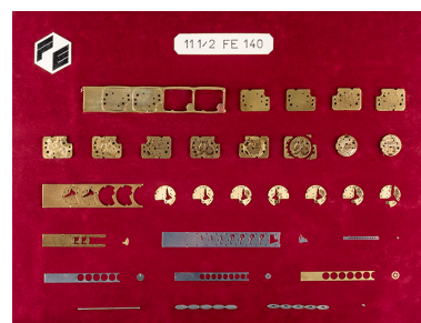
Phases de fabrication de composants d'un mouvement FE 140. (Collection musée de l'Horlogerie, Morteau). Phot. Sonia Dourlot IVR43_20192500297NUC4A
