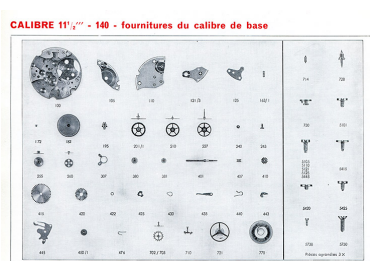
Calibre 11 1/2''' - 140 - fournitures du calibre de base, 1973. Autr. auteur inconnu IVR43_20162500135NUC2A
