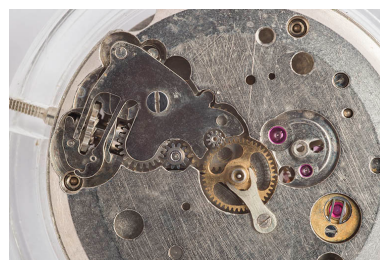
Mécanisme du remontoir (côté cadran). A droite, l'amortisseur de chocs. Phot. Sonia Dourlot IVR43_20152500008NUC4A
