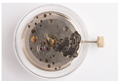
Vue d'ensemble, côté cadran. Phot. Sonia Dourlot IVR43_20152500006NUC4A
