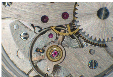
Détail : le balancier-spiral et son amortisseur de chocs (côté ponts). Le logo France Ebauches se devine en bas. Phot. Sonia Dourlot IVR43_20152500009NUC4A
