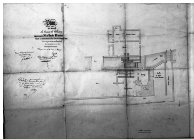
Plan de l'usine de Vellexon et des dépendances appartenant à Mr le Duc de Marmier [Plan- masse du haut fourneau]. Phot. Yves Sancey, Autr. Laumet IVR43_19877000087X
