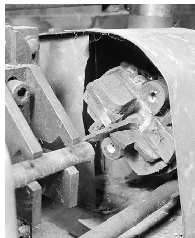
Détail de l'outil de coupe côté droit. Phot. Jérôme Mongreville IVR43_20022500500X
