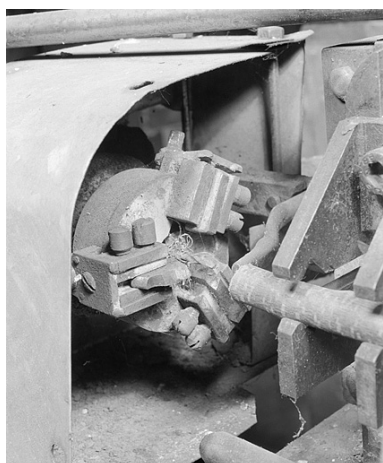
Détail de l'outil de coupe côté gauche. Phot. Jérôme Mongreville IVR43_20022500501X
