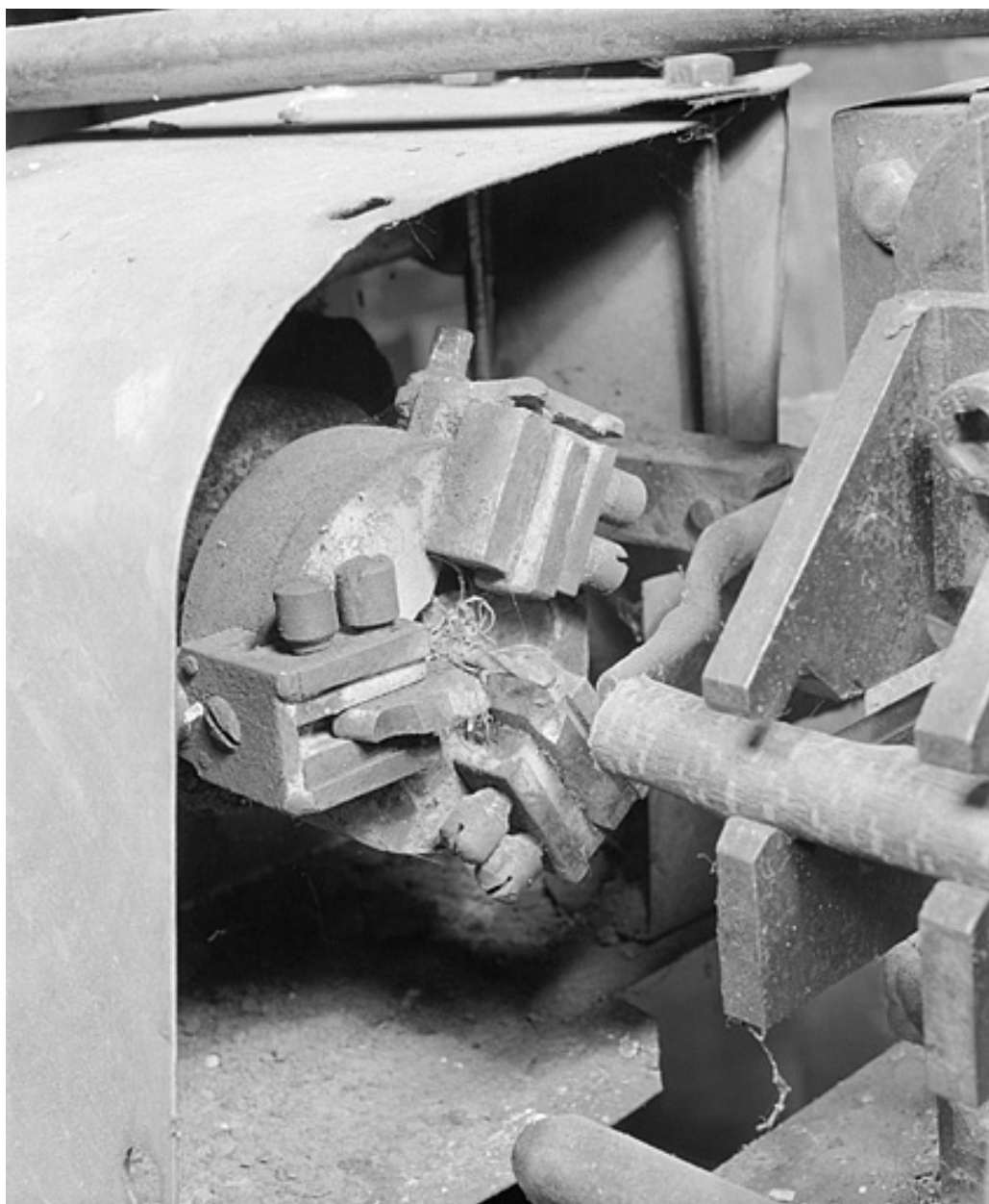
Détail de l'outil de coupe côté gauche.
