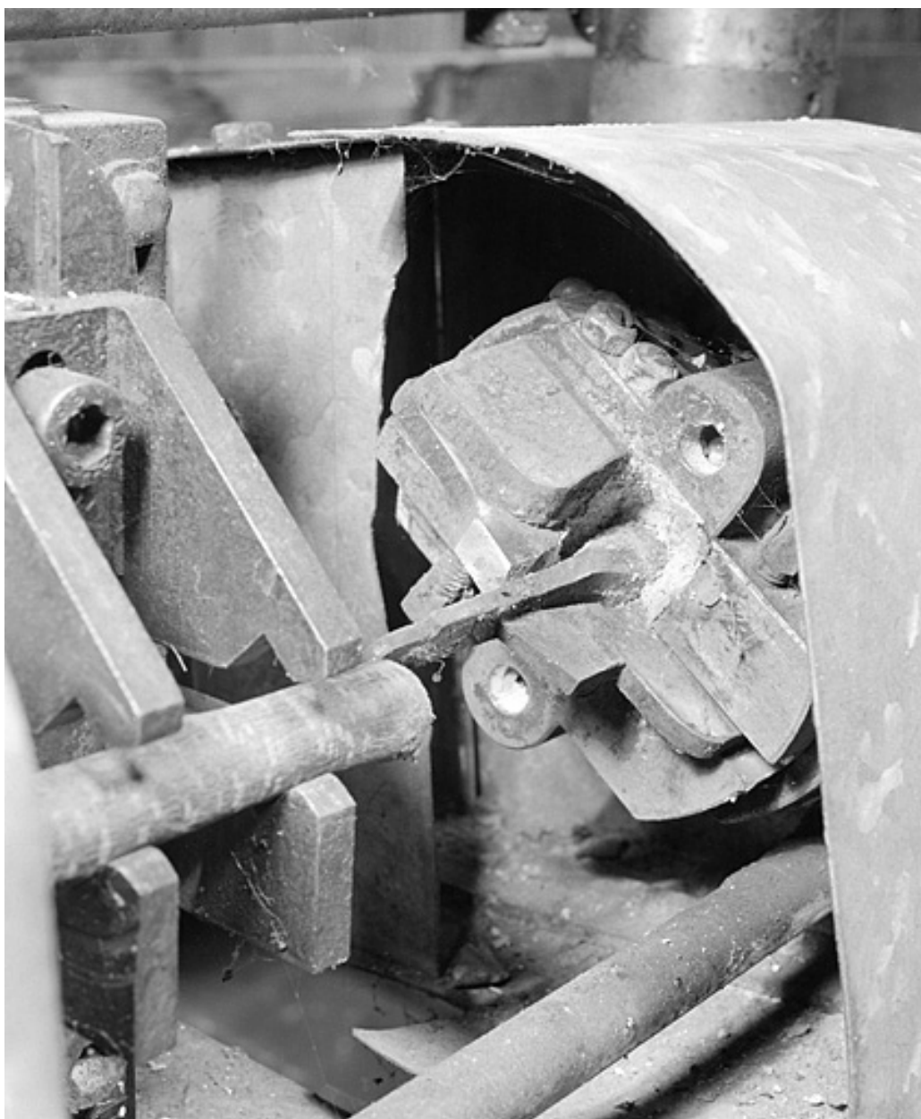
Détail de l'outil de coupe côté droit.
