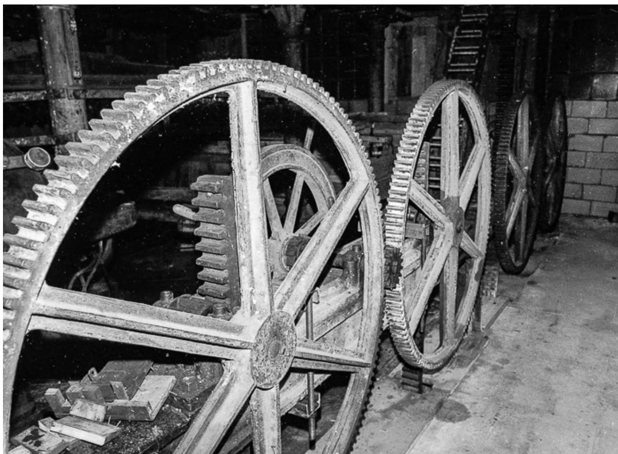
Eléments de transmission de la turbine en 1979.
