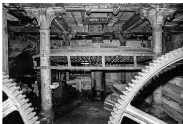
Mécanisme de transmission de la turbine (canal principal) en 1979. Phot. J. Dumont IVR43_19792501138Z
