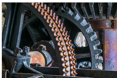
Rez-de-chaussée de l'atelier principal. Détail du mécanisme d'entraînement (engrenages coniques et roues dentées pour chaînes). Phot. Jérôme Mongreville IVR43_20152500386NUC4A
