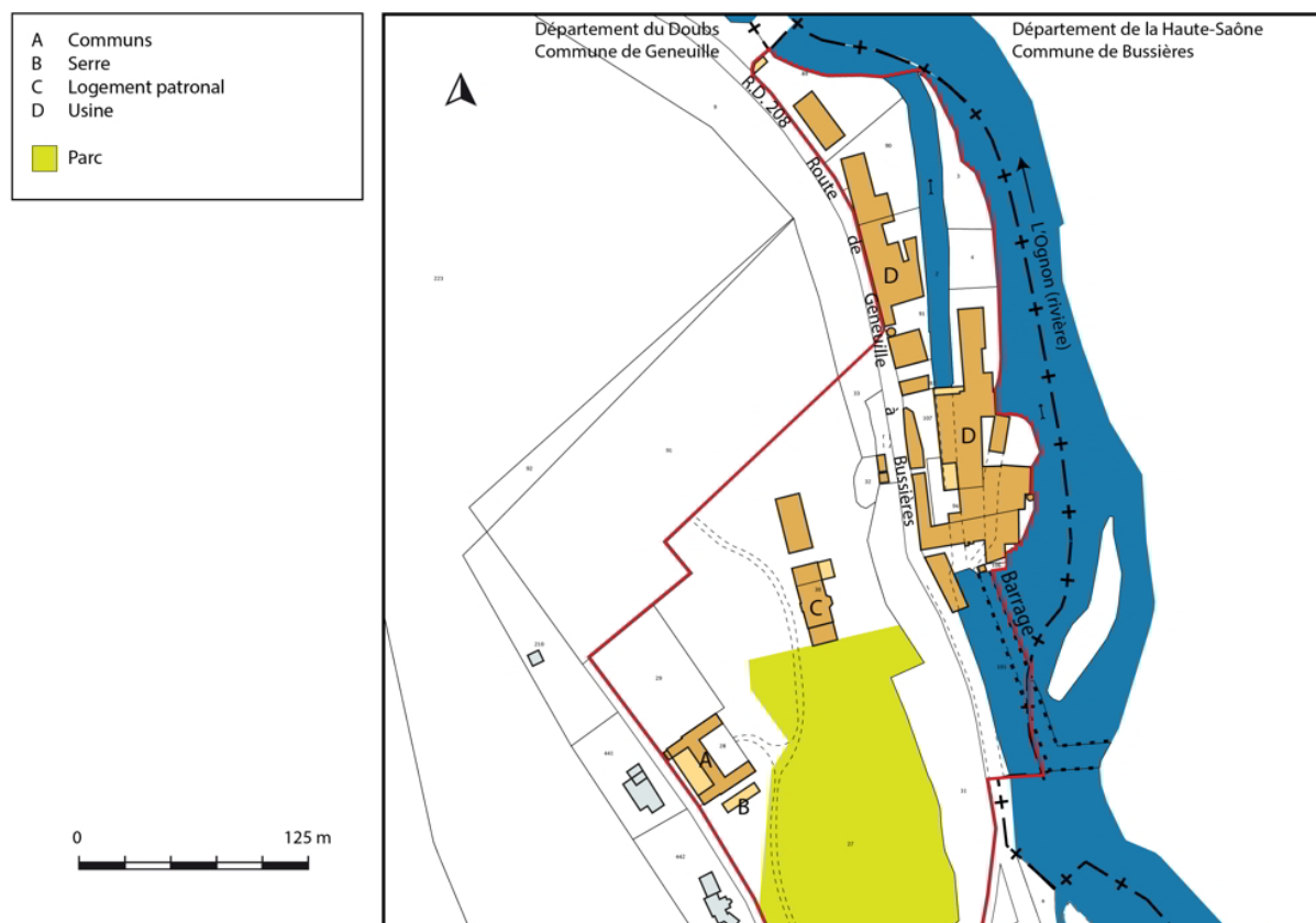
Plan de situation. Extrait du plan cadastral, 2019.
