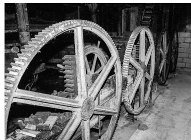
Eléments de transmission de la turbine en 1979. Phot. J. Dumont IVR43_19792501139Z
