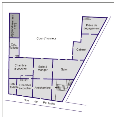
Croquis restituant la distribution intérieure du rez-de-chaussée au 18e siècle. Dess. André Céréza IVR43_20032500080NUDYY
