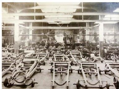
Châssis en cours de montage, phot. Stainacre, s.d. [début 20e siècle]. Phot. Stainacre IVR43_20162501110NUC4A
