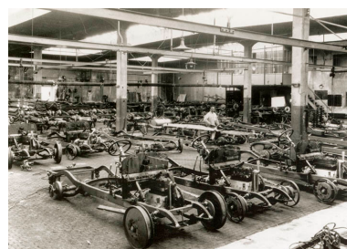
Atelier de montage. Châssis de véhicules, phot. Stainacre, s.d. [début 20e siècle]. Phot. Stainacre IVR43_20162501071NUC4A
