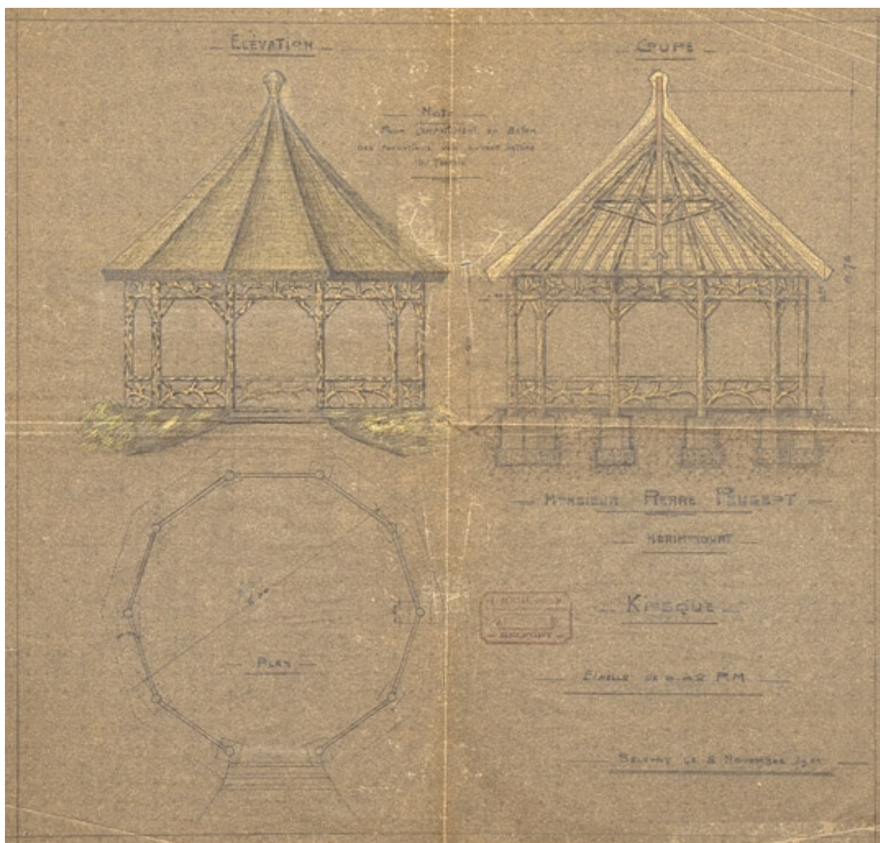
M. Pierre Peugeot. Hérimoncourt. Kiosque. Plan, coupe, élévation. Plan, calque, crayon, échelle 1/50, Belfort, novembre 1911.
