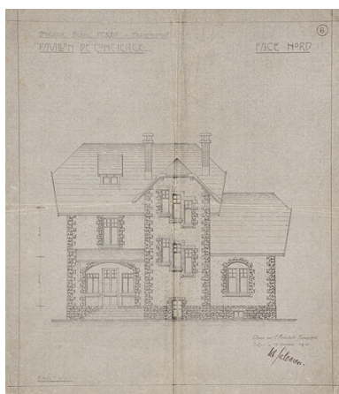
Propriété de M. Pierre Peugeot à Hérimoncourt. Pavillon de concierge. Face nord. Plan, calque, encre, échelle 1/50, Hérimoncourt, octobre 1910. Phot. Jérôme Mongreville, Autr. NEPASUTILISERSalomon Albert (architecte) IVR43_20122501164NUC4A
