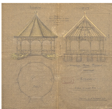
M. Pierre Peugeot. Hérimoncourt. Kiosque. Plan, coupe, élévation. Plan, calque, crayon, échelle 1/50, Belfort, novembre 1911. Phot. Jérôme Mongreville, Autr. NEPASUTILISERSalomon Albert (architecte) IVR43_20122501163NUC4A
