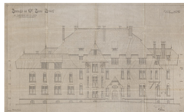
Propriété de M. Pierre Peugeot à Hérimoncourt. Face sud. Plan, calque, encre, échelle 1/50, Hérimoncourt, mai 1910. Phot. Jérôme Mongreville, Autr. NEPASUTILISERSalomon Albert (architecte) IVR43_20122501161NUC4A
