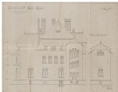
Propriété de M. Pierre Peugeot à Hérimoncourt. Face est. Plan, calque, encre, échelle 1/50, Hérimoncourt, mai 1910. Phot. Jérôme Mongreville, Autr. NEPASUTILISERSalomon Albert (architecte) IVR43_20122501159NUC4A
