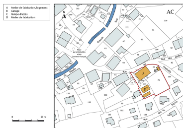
Plan-masse et de situation. Extrait du plan cadastral, 2017, section AC, 1/1 000. Dess. Mathias Papigny IVR43_20172501269NUDA
