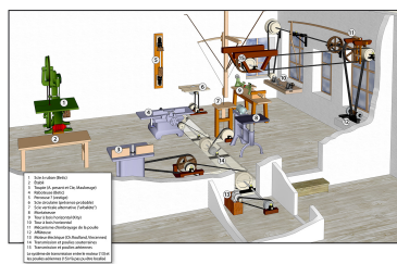
Plan de disposition des machines à l'étage de soubassement. Dess. Mathias Papigny IVR43_20162501771NUDAQ
