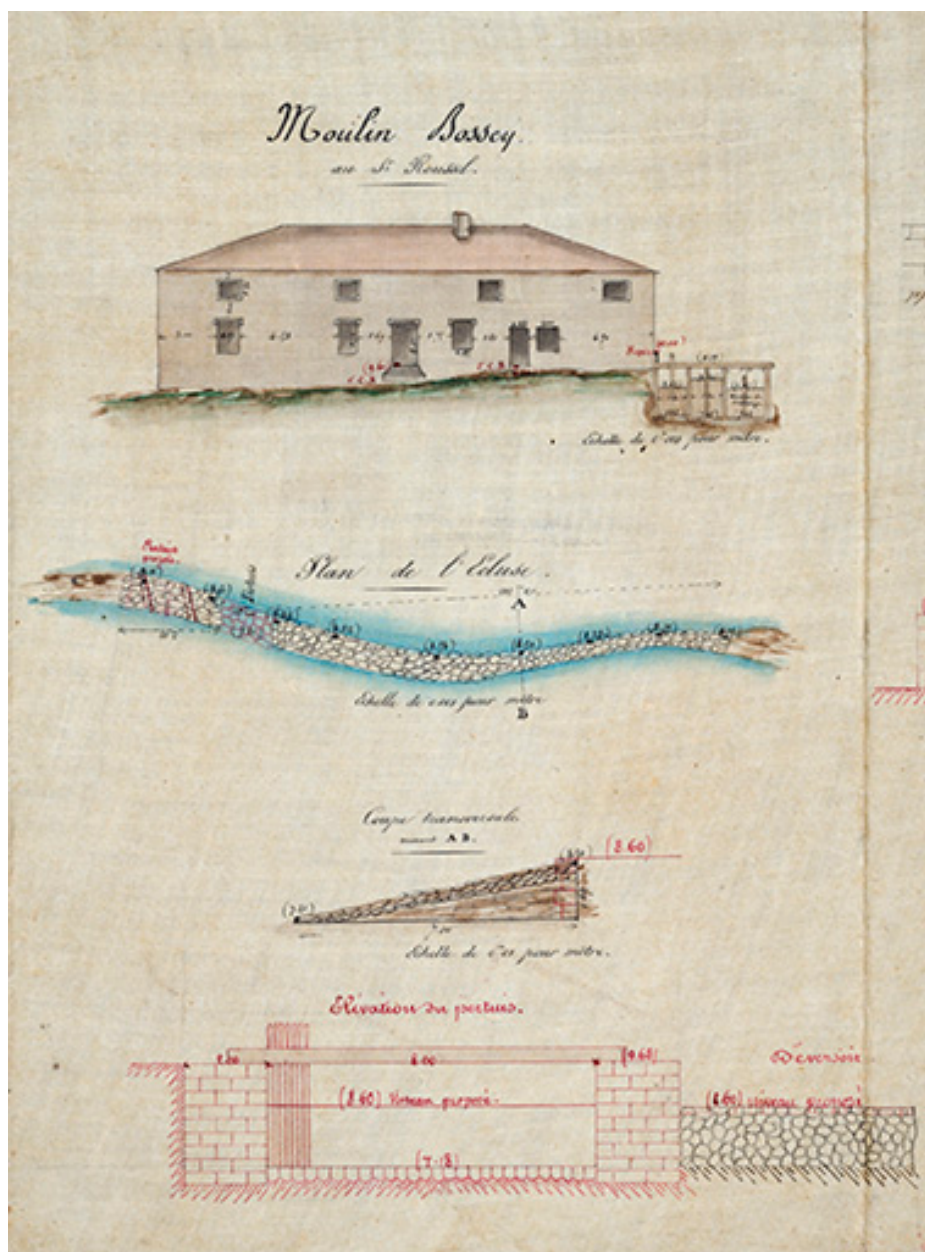
Plan du moulin Bossey (1857).
