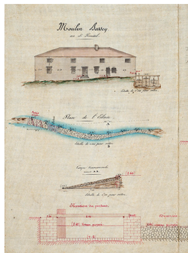
Plan du moulin Bossey (1857). Phot. Jérôme Mongreville, Autr. auteur inconnu IVR43_20167001571NUC4A
