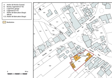
Plan-masse et de situation. Extrait du plan cadastral, 2019, section D. Dess. Bertrand Turina IVR43_20202500306NUDA
