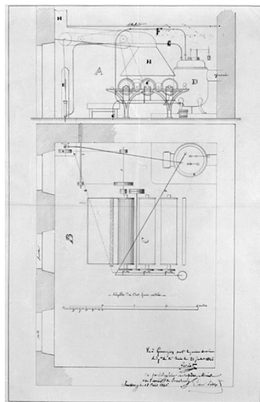
Plan de l'atelier de parage.
