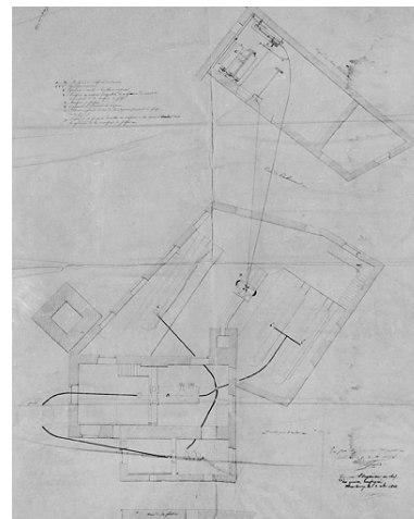
Plan de situation de la salle des machines à vapeur.
