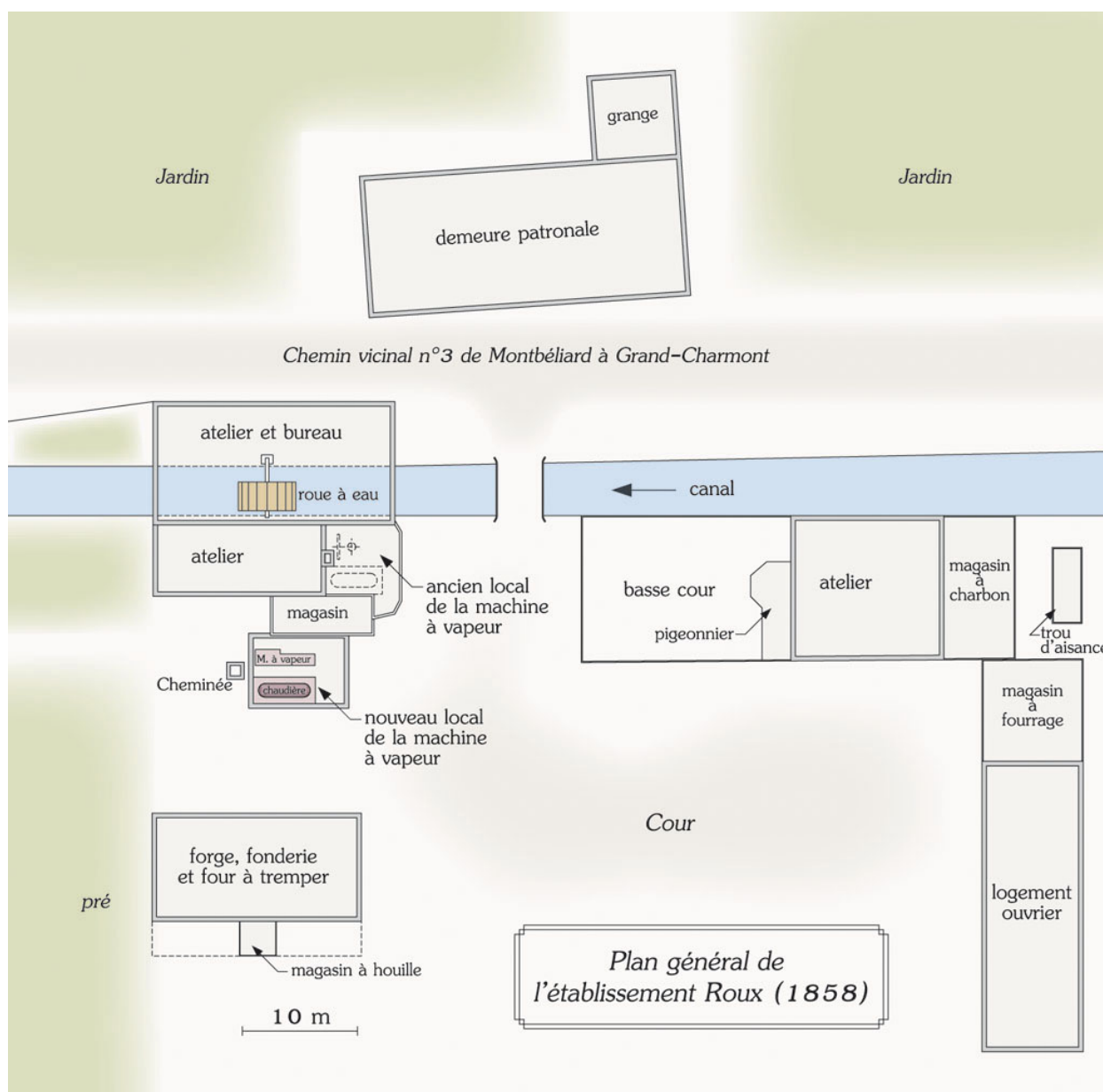
Plan général de l'usine d'horlogerie Roux, dessin. D'après un calque de 1858, échelle 1/100, conservé aux AD Doubs (432 S 6).
