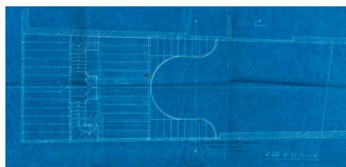
[Plans et coupes du cinéma projeté pour Henri Botex]. Premières. S.d. [1909]. Phot. Pierre-Marie Barbe- Richaud, Autr. Adrien Lelièvre IVR26_20238900838NUC2A
