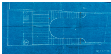
[Plans et coupes du cinéma projeté pour Henri Botex]. Deuxièmes. S.d. [1909]. Phot. Pierre-Marie Barbe- Richaud, Autr. Adrien Lelièvre IVR26_20238900839NUC2A
