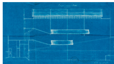
[Plans et coupes du cinéma projeté pour Henri Botex]. Coupe suivant l'axe. S.d. [1909]. Phot. Pierre-Marie Barbe- Richaud, Autr. Adrien Lelièvre IVR26_20238900837NUC2A
