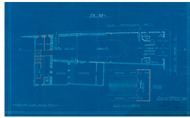
Select Cinéma [...] Projet de transformation de l'entrée et aménagement de WC et de cabine. [Détail : ] Plan. 26 août 1931. Phot. Pierre-Marie Barbe-Richaud, Autr. Jacques Agénie IVR26_20238900834NUC4A
