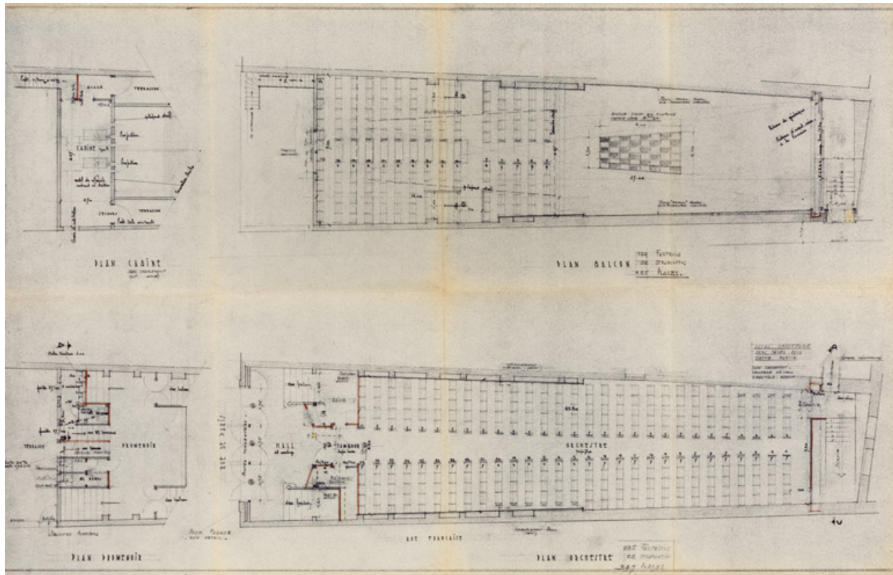
Cinéma « Le Select ». Rue de Paris. Auxerre. Yonne. Projet de transformation. Plans. 9 mai 1958.
