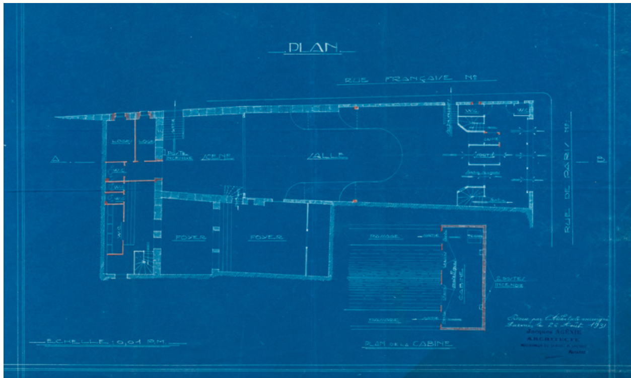
Select Cinéma [...] Projet de transformation de l'entrée et aménagement de WC et de cabine. [Détail : ] Plan. 26 août 1931.
