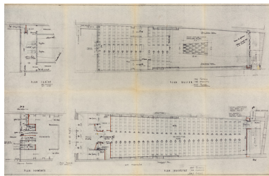
Cinéma « Le Select ». Rue de Paris. Auxerre. Yonne. Projet de transformation. Plans. 9 mai 1958. Phot. Pierre-Marie Barbe-Richaud, Autr. Lucien Thomas IVR26_20238900831NUC4A
