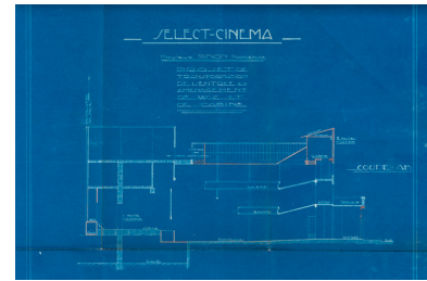
Select Cinéma [...] Projet de transformation de l'entrée et aménagement de WC et de cabine. [Détail : ] Coupe. 26 août 1931. Phot. Pierre-Marie Barbe-Richaud, Autr. Jacques Agénie IVR26_20238900835NUC4A
