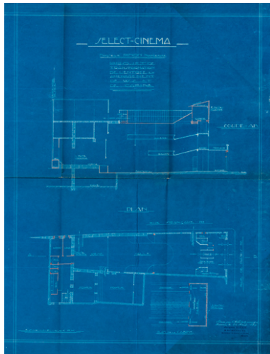
Select Cinéma [...] Projet de transformation de l'entrée et aménagement de WC et de cabine. 26 août 1931. Phot. Pierre-Marie Barbe-Richaud, Autr. Jacques Agénie IVR26_20238900833NUC2A
