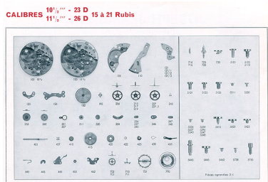
Calibres [jeambrun] 10 1/2''' - 23 D D [et] 11 1/2''' - 26 D - 15 à 21 rubis [éclaté des fournitures], 1973.
