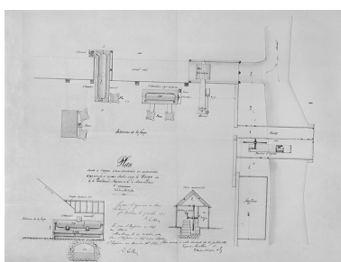
Plan dressé à l'appui d'une demande en autorisation d'appareils à vapeur établis dans la forge de MM.
