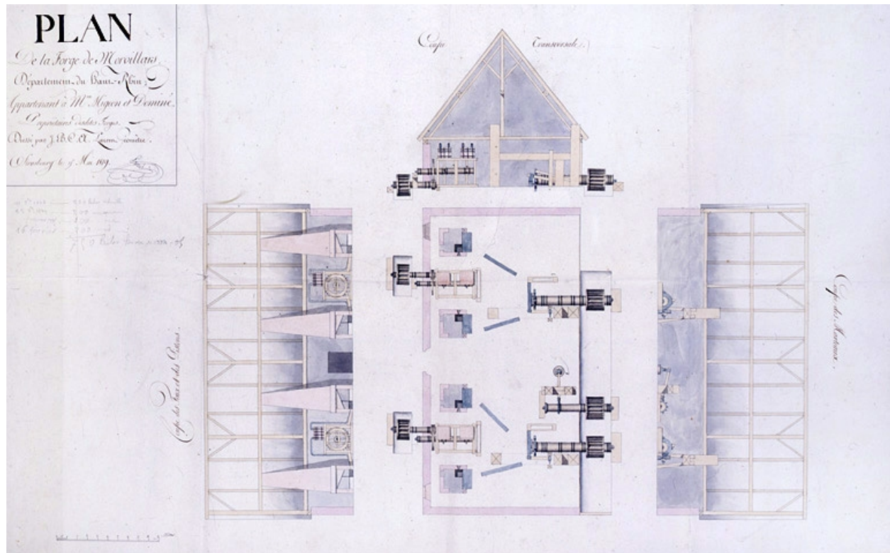
Plan de la forge de Morvillars [...]. Coupe des marteaux, coupe transversale, coupe des feux et des pistons.
