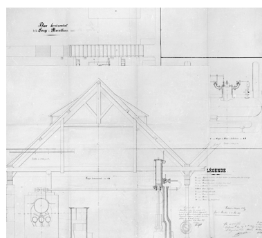
Plan horizontal de la forge de Morvillars (1857) [coupe transversale de la chaudière].
