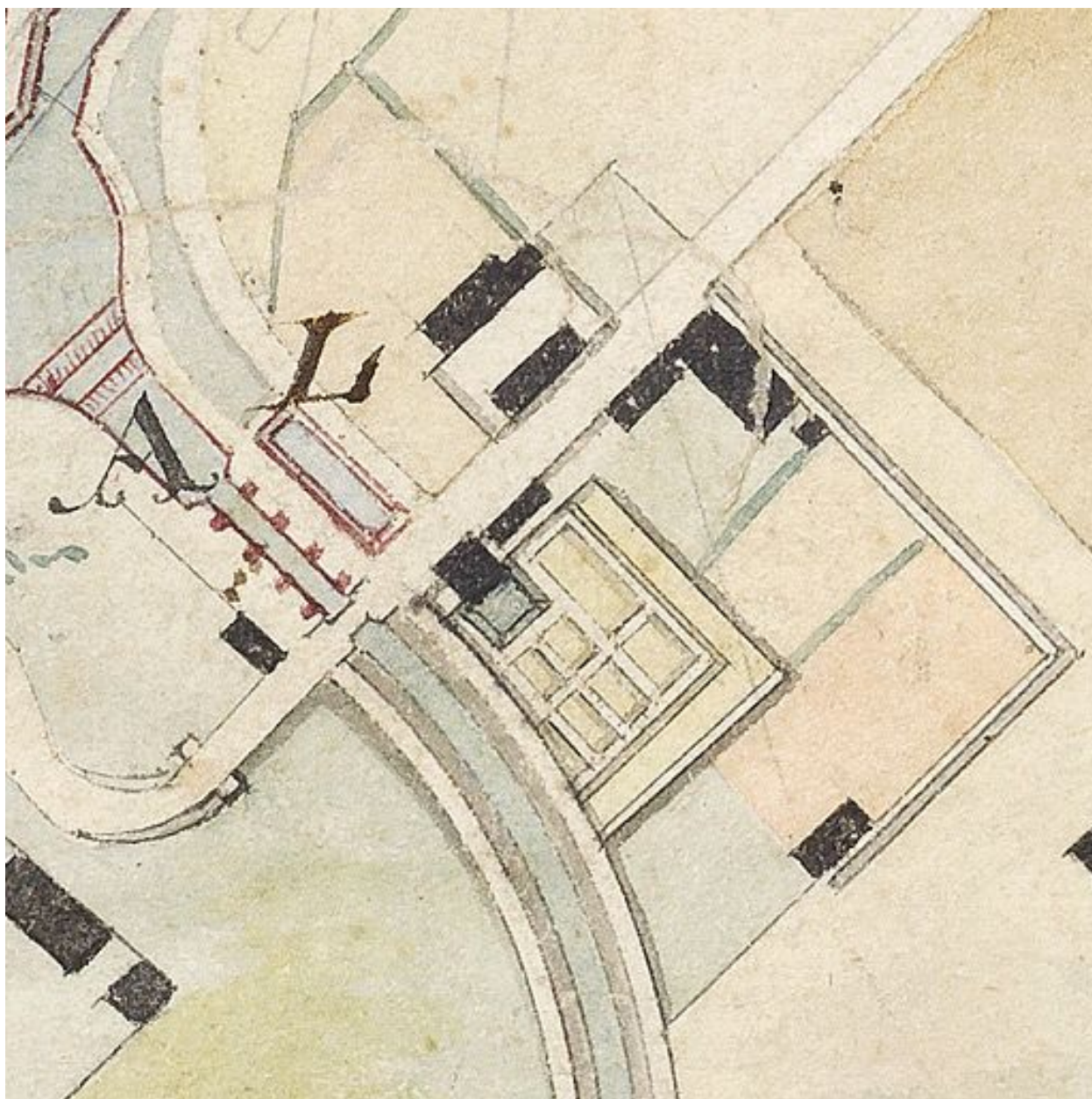
"Carte topographique des différents étangs destinés à former le réservoir du point de partage du Canal du Nivernais" : détail du pavillon des ingénieurs et des jardins. (Archives VNF-direction territoriale Centre-Bourgogne ; subdivision de Corbigny)
