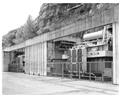
Vue d'ensemble des transformateurs. Phot. Jérôme Mongreville IVR43_19913900697V
