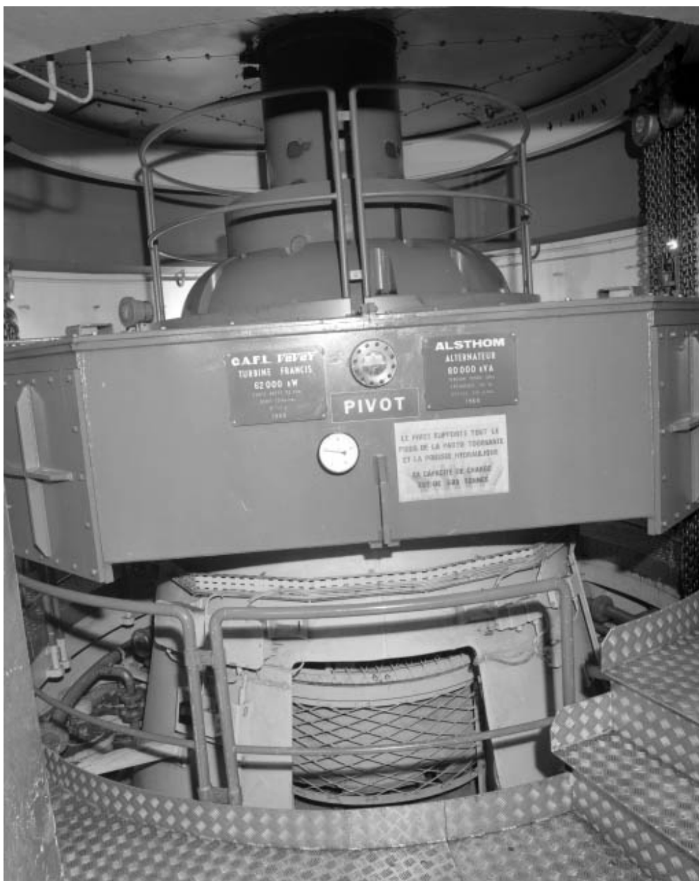
Pivoterie du premier groupe (cadre vertical).
