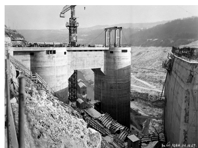
Prise d'eau. Phot. Jérôme Mongreville, Autr. Studios Villeurbannais Monchanin et Périchon IVR43_19913900317X
