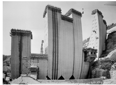
Barrage - Vue d'ensemble des plots PQ à CD - Vue de l'amont. Phot. Jérôme Mongreville, Autr. Studios Villeurbannais Monchanin et Périchon IVR43_19913900312X
