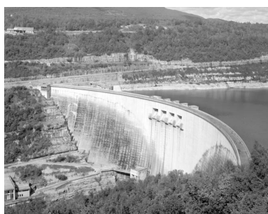
Le barrage, depuis l'est. Phot. Jérôme Mongreville IVR43_19913900669X
