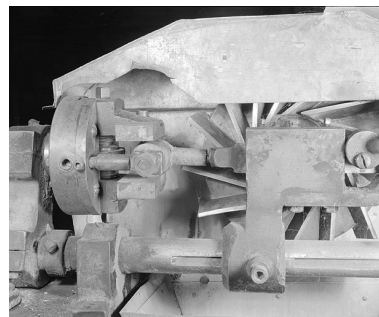
Le mandrin "gueule de loup". Phot. Jérôme Mongreville IVR43_20022500601X
