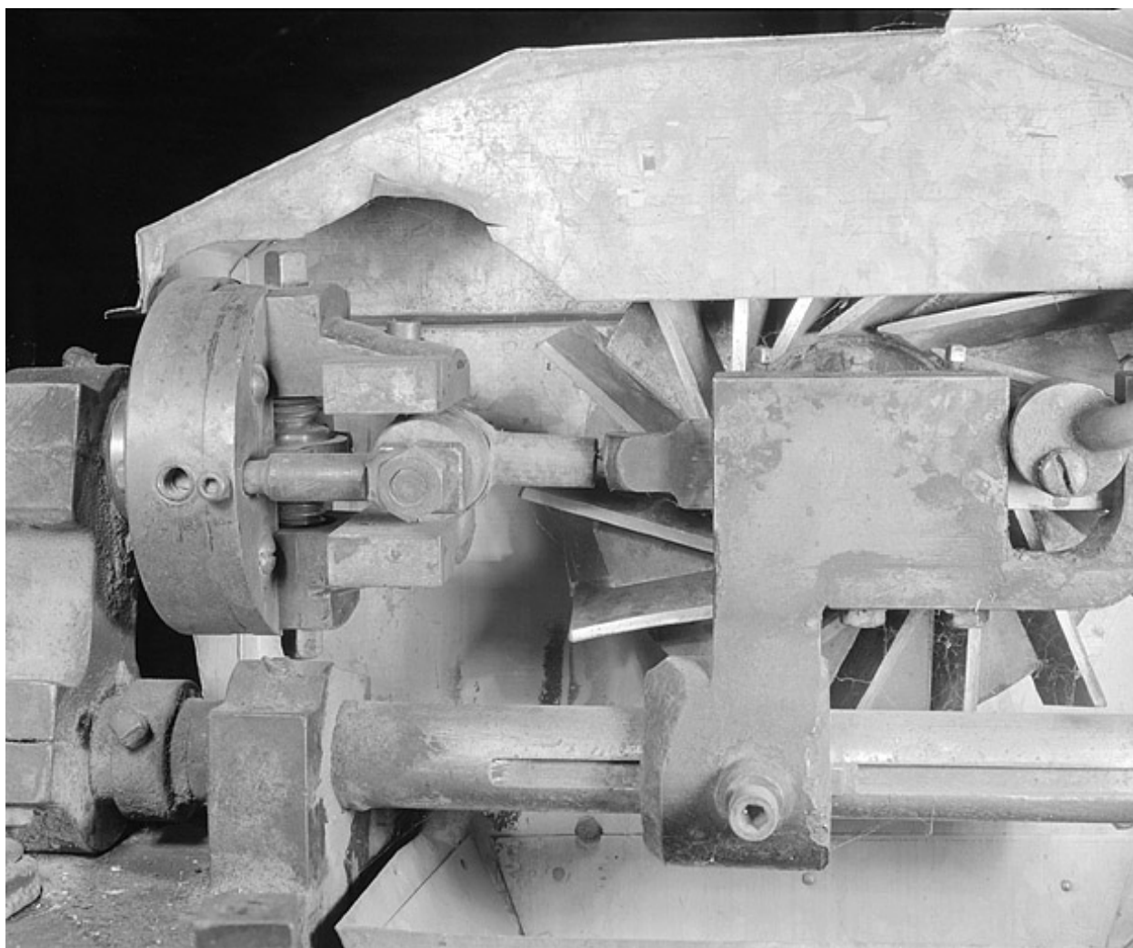
Le mandrin "gueule de loup".
