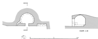
Plan. et coupe A-B Dess. Alain Morelière IVR26_20122100521A3YY
