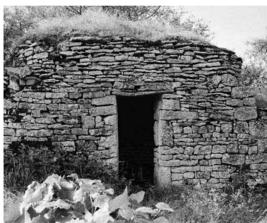
Vue de l'élévation antérieure de la cabane. Phot. Jean-Luc Duthu IVR26_19802100875X
